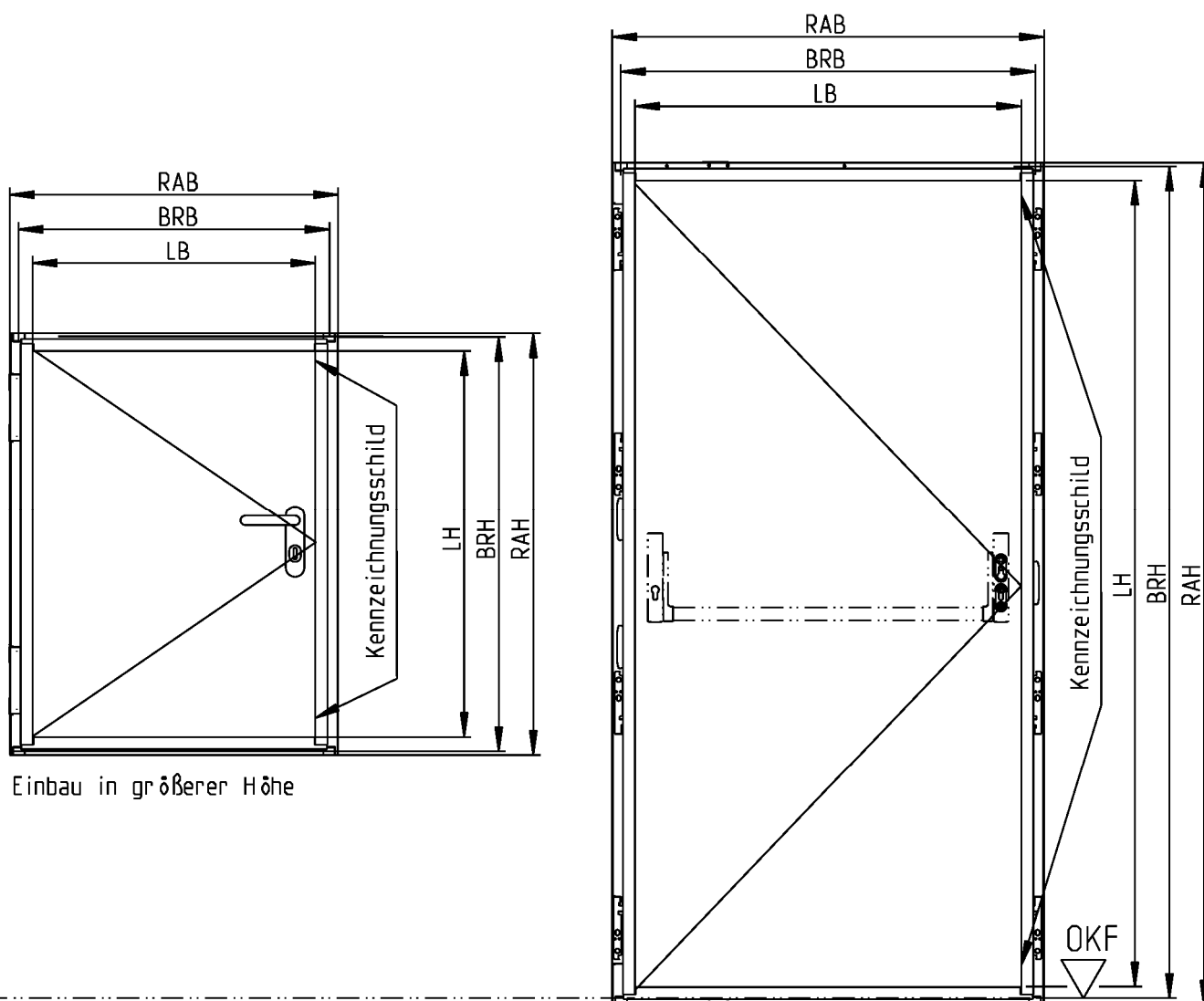
Ansicht Schließseite
