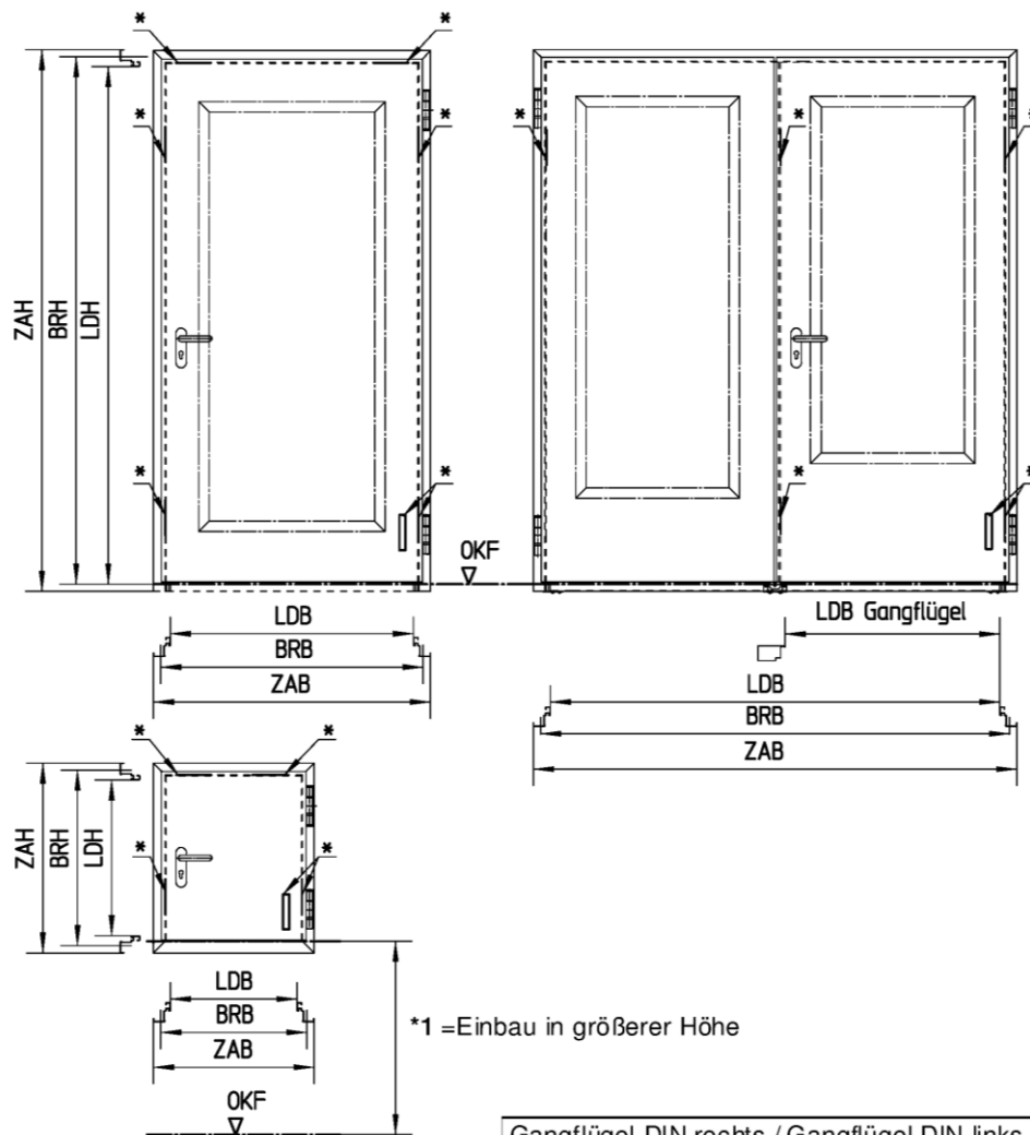
Gangflügel DIN rechts / Gangflügel DIN links spiegelbildlich
