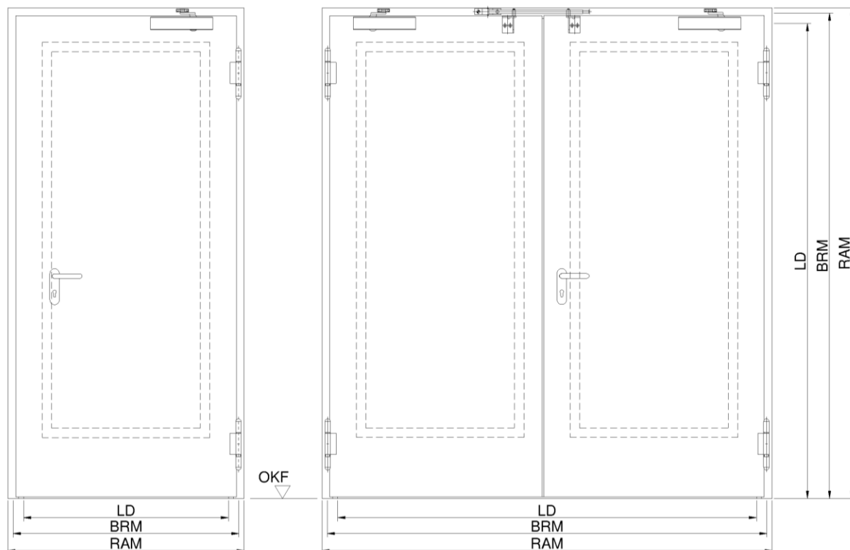
dargestellt: Anschlagrichtung DIN Rechts, DIN Links spiegelbildlich
