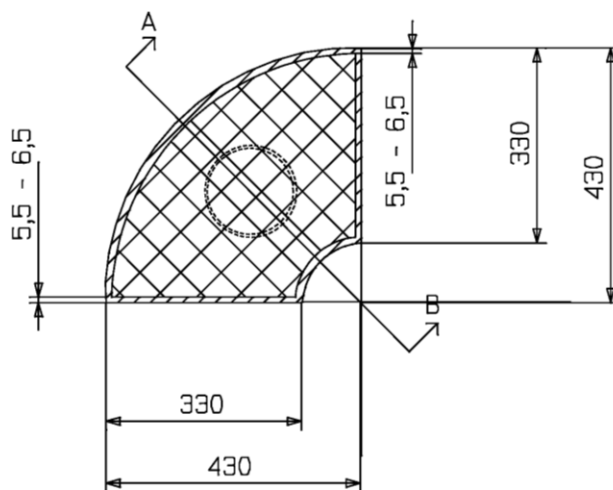
Schnitt A-B
