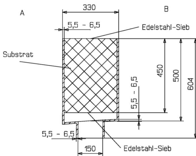
Schnitt A-B
