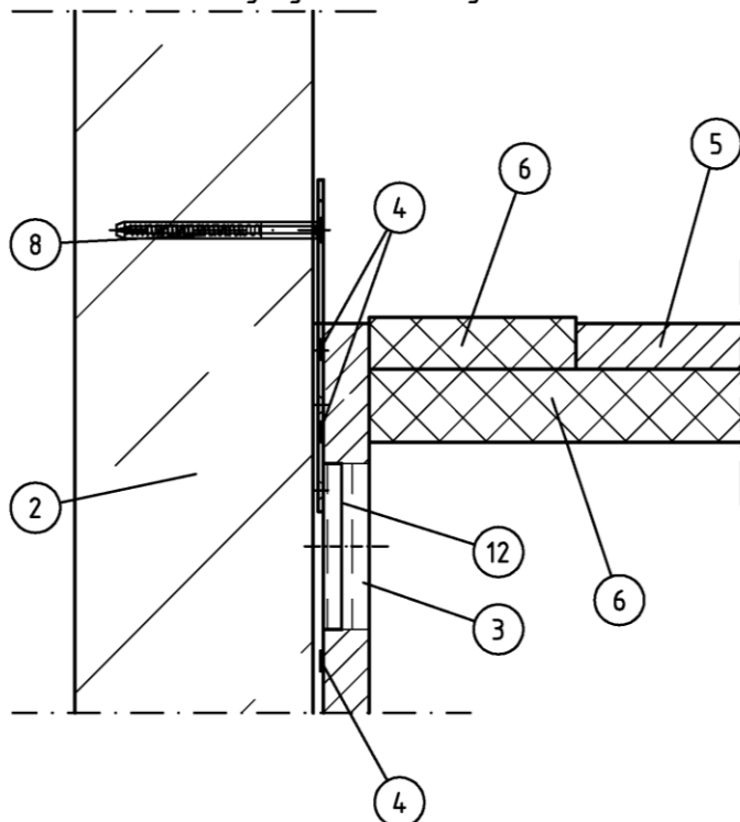
Detail B Kabeleinführung unten
