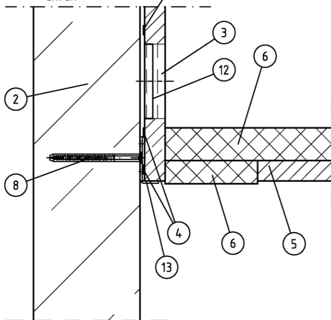
Detail B Kabeleinführung unten
