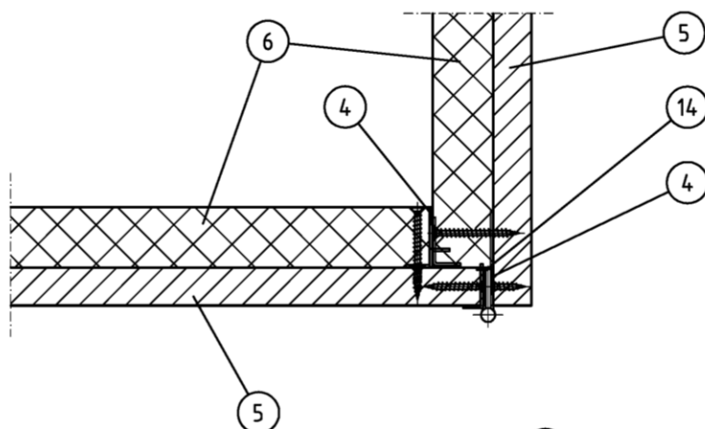
Detail Kabeleinführung
