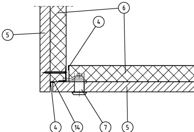
Detail D Bandseite
