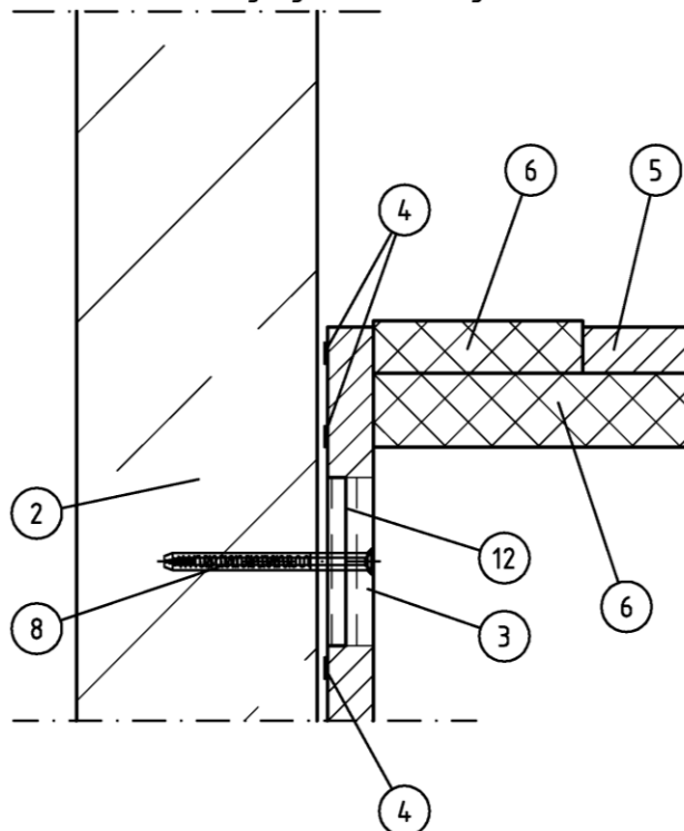
Detail A ESL Kabeleinführung oben und Befestigung Brandschutzgehäuse
