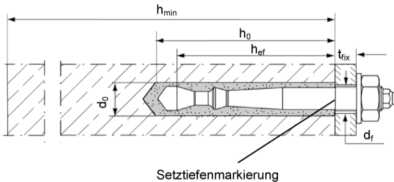
Highbond- Anker FHB II - A S Vorsteckmontage und Durchsteckmontage
