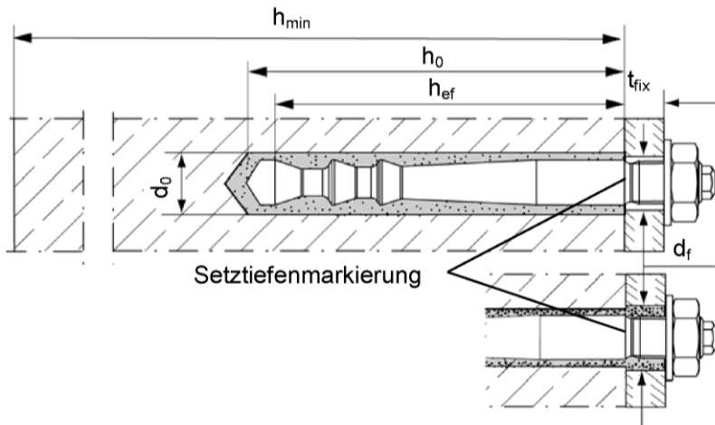
Highbond- Anker FHB II - A L Vorsteckmontage
