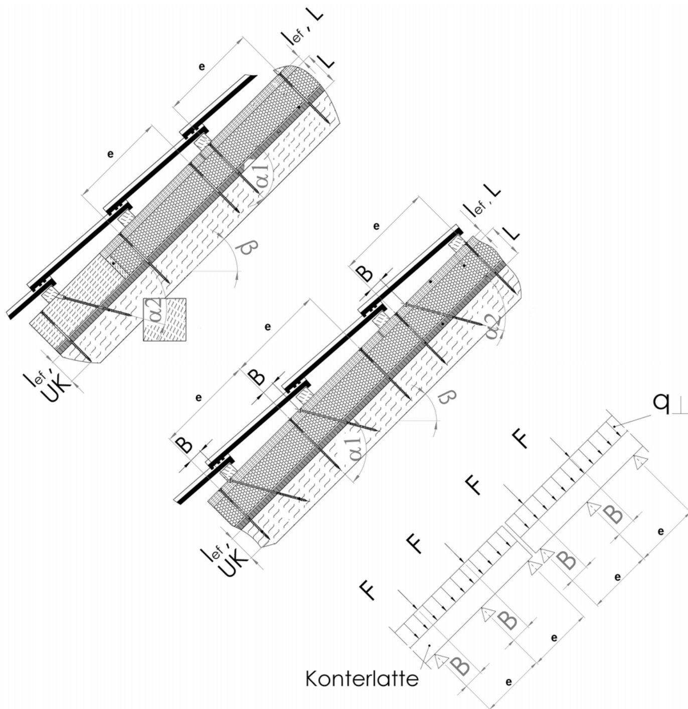
Abbildung A.5.4: Befestigung der Aufdach-Dämmung auf Sparren – Prinzipdarstellung mit wechselnder Neigung angeordneter Schrauben und durchlaufende Konterlatte beansprucht aus konstanter Linienlast auf die Dachfläche q_{\perp} und Einzellasten aus den zugbeanspruchten Schrauben F_{Zs}
