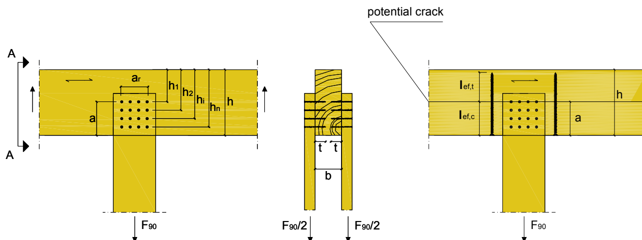
Abbildung 4.1: Beispiel für die Verstärkung eines Queranschlusses
