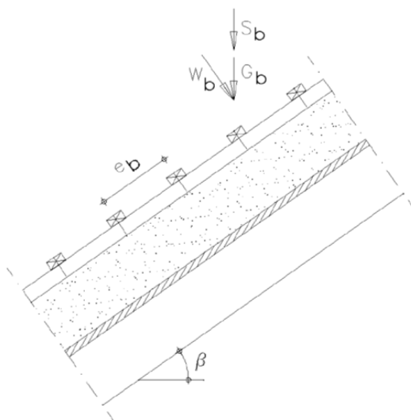
Abbildung A.5.2: Einzellasten F_b rechtwinklig zu den Konterlatten
