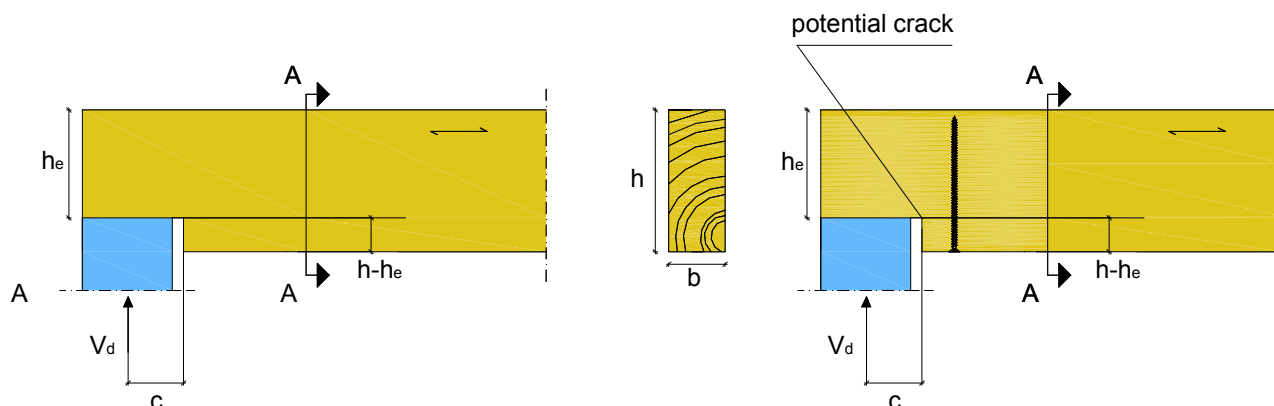
Abbildung 4.2: Beispiel für die Verstärkung einer Ausklinkung bei Zugbeanspruchung rechtwinklig zur Faser
