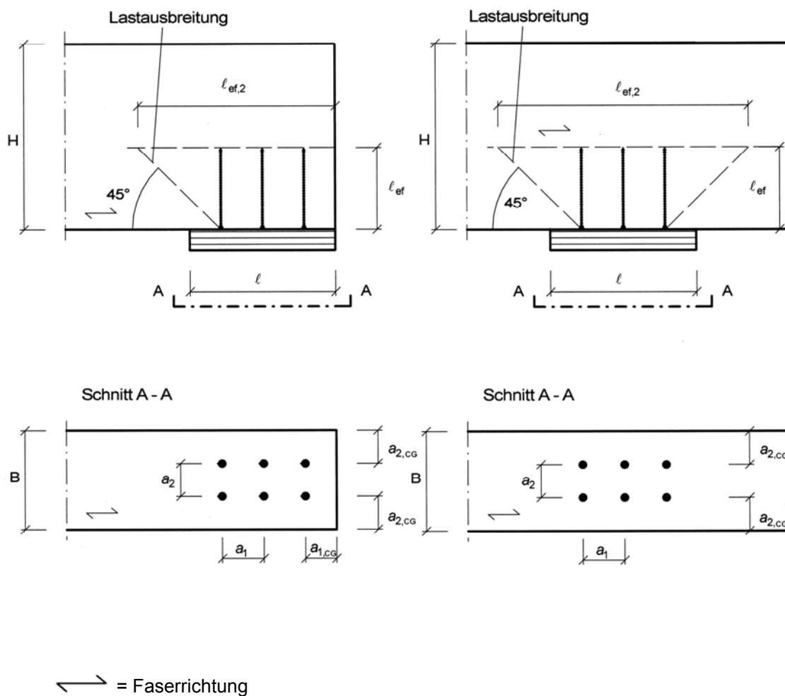
Abbildung 3.1: Verstärktes Endauflager (links) und verstärktes Zwischenauflager (rechts)
