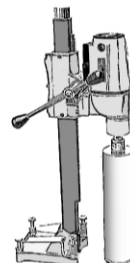
Diamantbohrkronen (DD)
