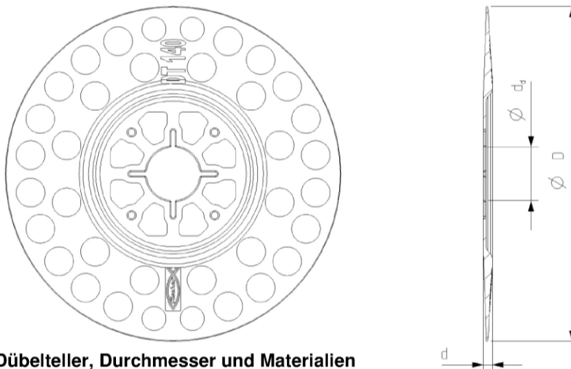
Zeichnung der Dübelteller
