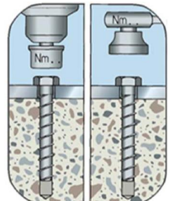
Schraube eindrehen
