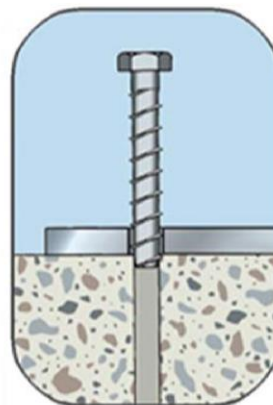
Schraube setzen
