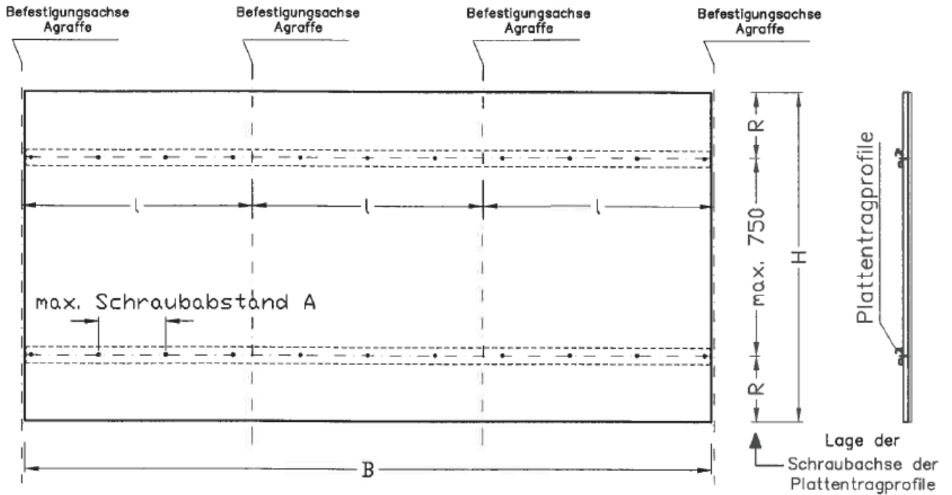
liegende Paneelanordnung für maximale Plattenformate (BxH) 2600mm x 1250mm Alle Maße in mm
