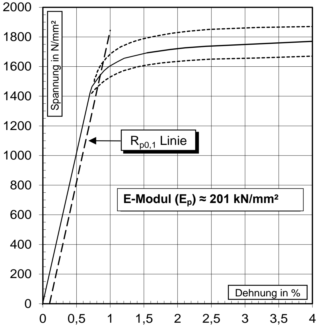
Bild 2: Spannungs - Dehnungslinie
