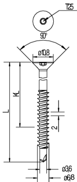
JT3-ST-2-6,8 x L JT2-ST-2-6,8 x L
