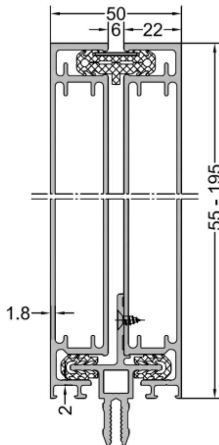
Montagepfosten
