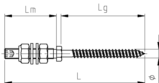
Für Holz - Unterkonstruktion SP - A 8,4 / M8 x L SP - A 8,4 / M10 x L
