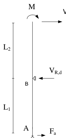
Abb. 4: Statisches System der Solarbefestiger
