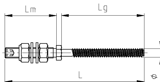
Für Stahl - Unterkonstruktion SP - BZ 8,0 / M8 x L SP - BZ 8,0 / M10 x L
