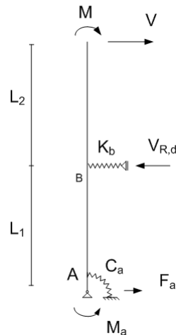
Abb. 5: Statisches System für das alternative Nachweisverfahren der Querkrafttragfähigkeit
