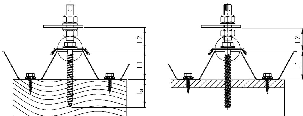
Abb. 1: Befestigung der benachbarten Wellentäler bei Holz- bzw. Stahlunterkonstruktionen
