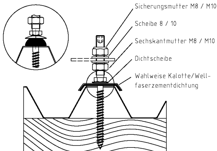
Auf Holz - Unterkonstruktion SP - A 8,4 / M8 x L SP - A 8,4 / M10 x L
