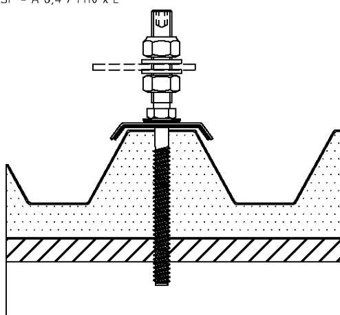
Auf Stahl - Unterkonstruktion SP - BZ 8,0 / M8 x L SP - BZ 8,0 / M10 x L
