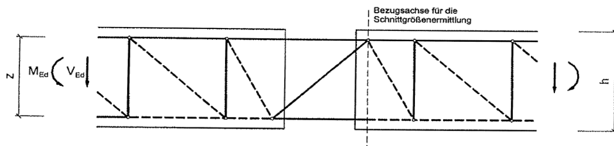
IPT indirekte Stützung
