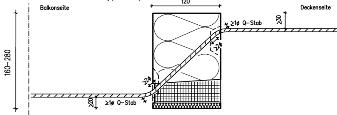
Ansicht Balkonseite
