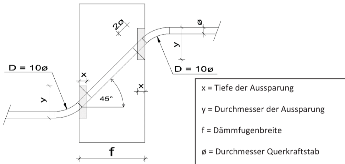
Abb. 12: Regelung Querkraftstab im Bereich der Fuge
