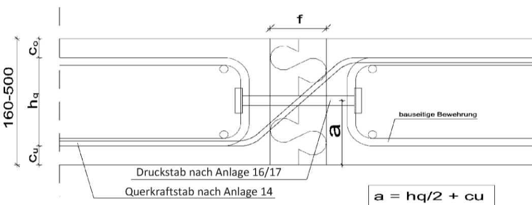
Abb. 5: Egcobox Typ PV – mittiger Druckstab
