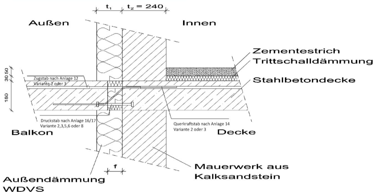
Abb. 47: Einbausituation mit Lagerung an gegenüberliegenden Rändern
