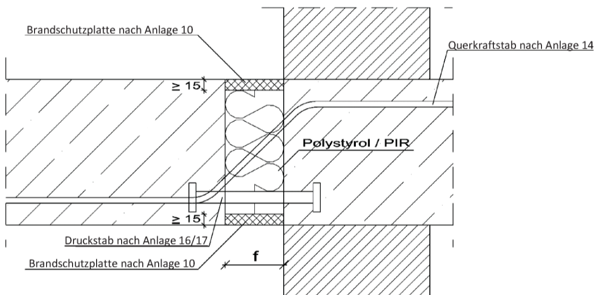
Abb. 29: Egibox Typ PV (Brandschutz)
