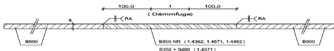
Abb. 22: Druckstabvariante 3
