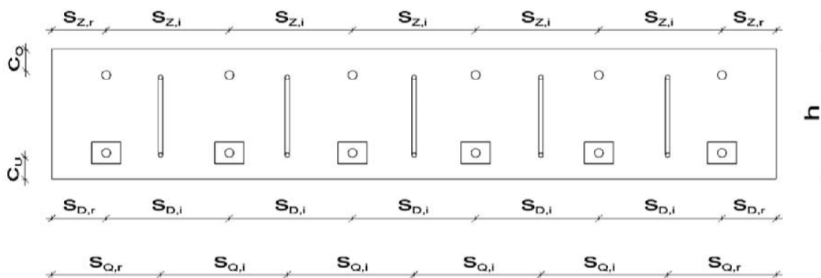
Abb. 13: Geometrische Randbedingungen
