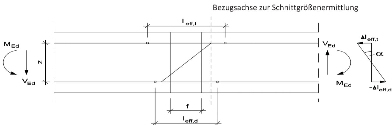
Abb. 43: Modell zur Ermittlung der Biegeverformung in der Fuge
