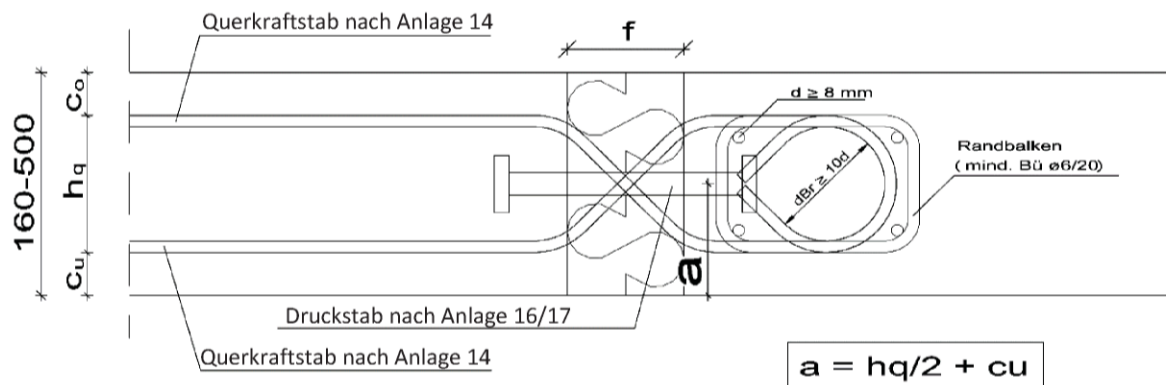
Abb. 11: Egobox Typ PV± – mittiger Druckstab
