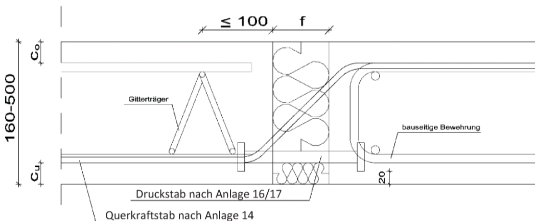
Abb. 4: Egcobox Typ PV
