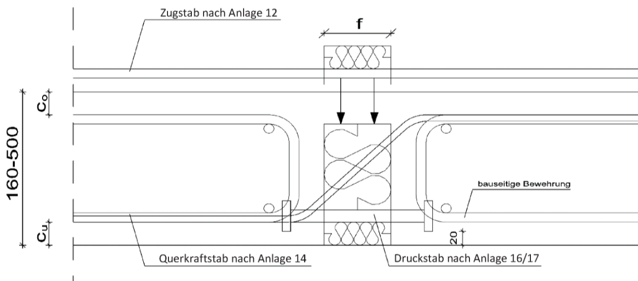
Abb. 2: Egobox Typ P-F
