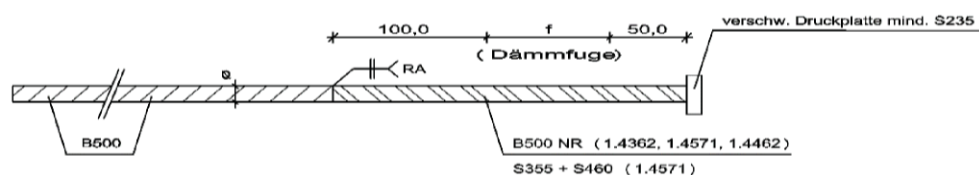
Abb. 25: Druckstabvariante 6
