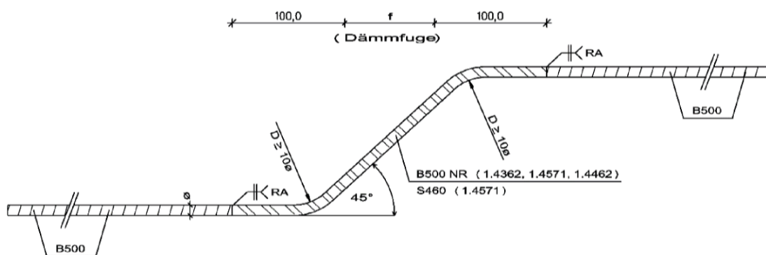
Abb. 19: Querkraftstabvariante 3
