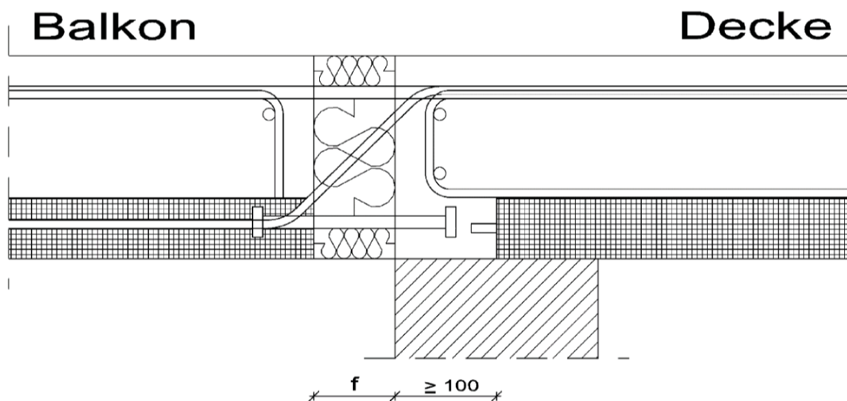
Abb. 44: Beispiel in Elementdecken - Bügel auf dem Elementdeckenspiegel
