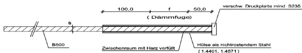
Abb. 23: Druckstabvariante 4
