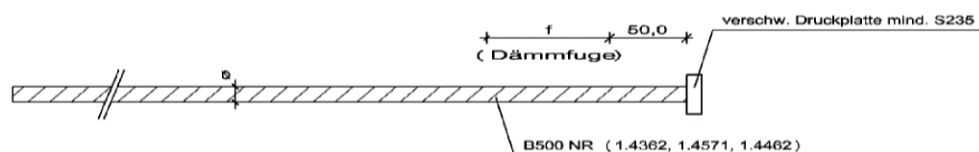
Abb. 24: Druckstabvariante 5
