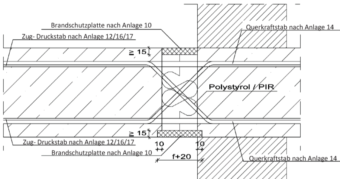
Abb. 32: Egibox Typ P± (Brandschutz)
