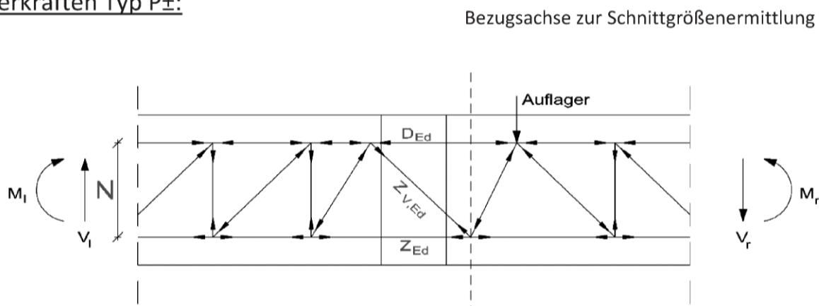
Abb. 38: Egcobox Typ P± (statisches System)
