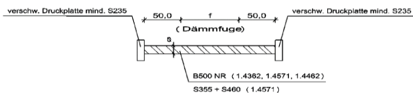
Abb. 27: Druckstabvariante 8
