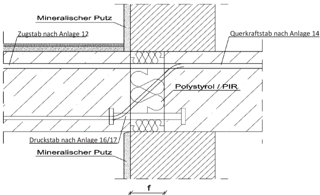
Abb. 34: Egibox Typ P (Brandschutz)
