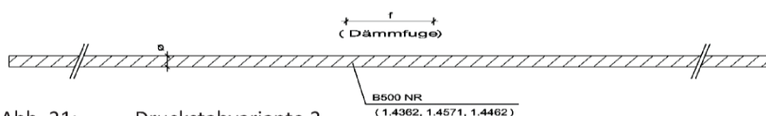
Abb. 21: Druckstabvariante 2
