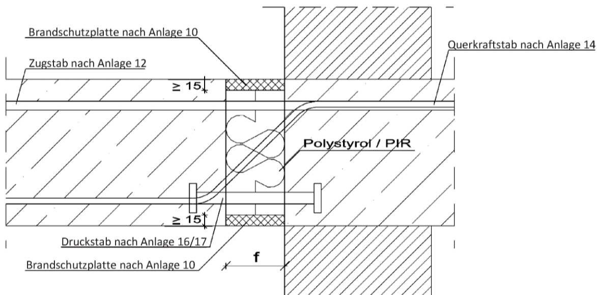
Abb. 28: Egibox Typ P (Brandschutz)
