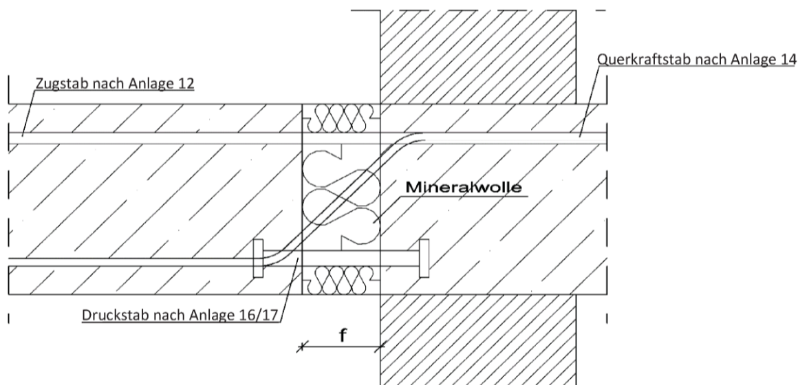
Abb. 30: Egibox Typ P (Brandschutz)
