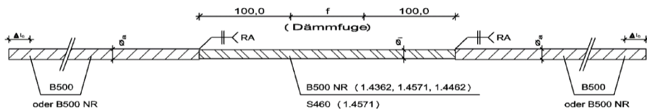
Abb. 16: Zugstabvariante 3
