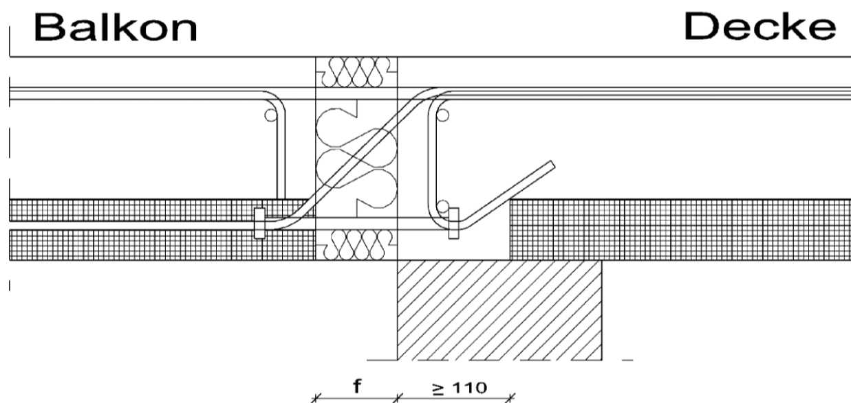
Abb. 45: Beispiel in Elementdecken - Bügel gekröpft
