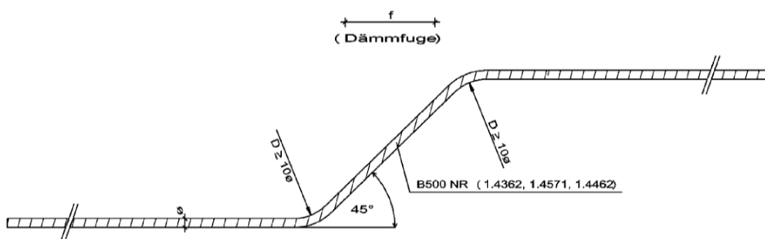
Abb. 18: Querkraftstabvariante 2
