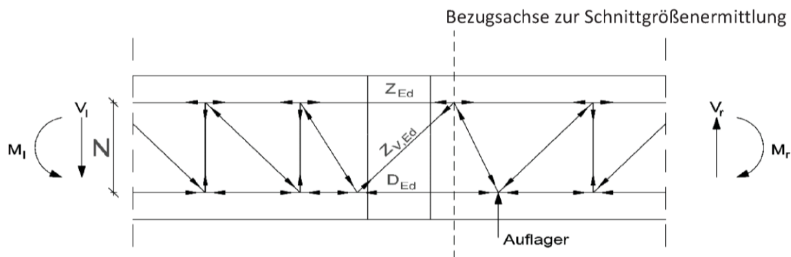
Abb. 36: Egcobox Typ P (statisches System)
