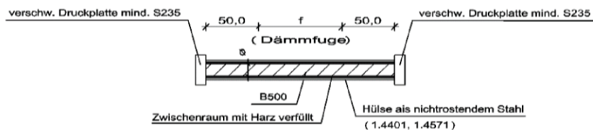
Abb. 26: Druckstabvariante 7
