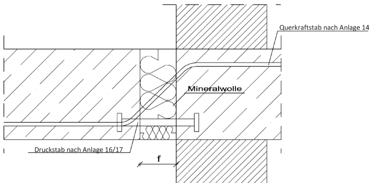
Abb. 31: Egibox Typ PV (Brandschutz)
