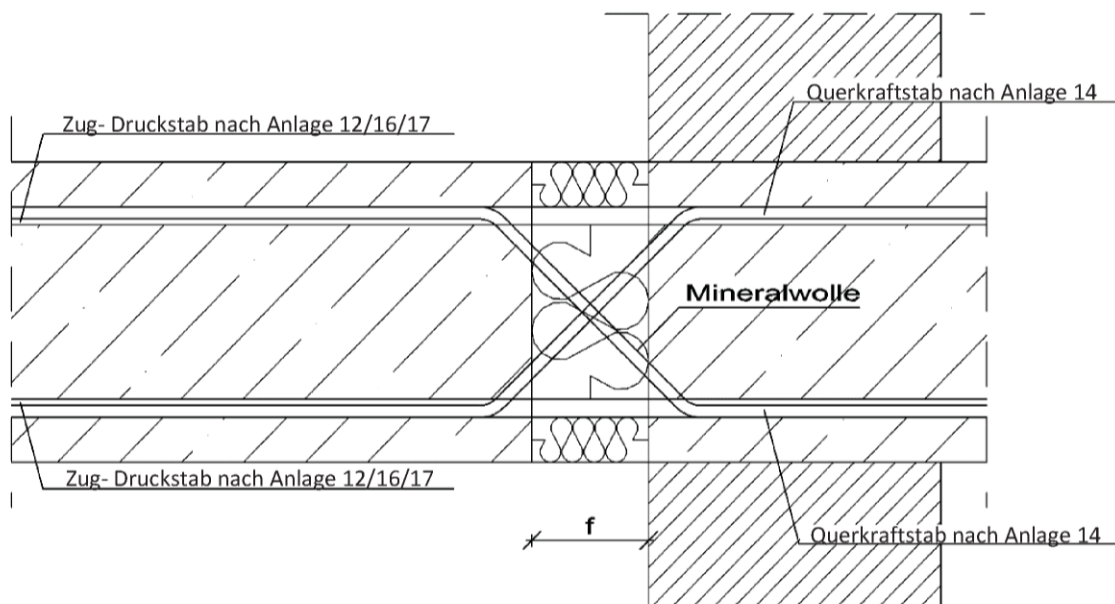
Abb. 33: Egibox Typ P± (Brandschutz)
