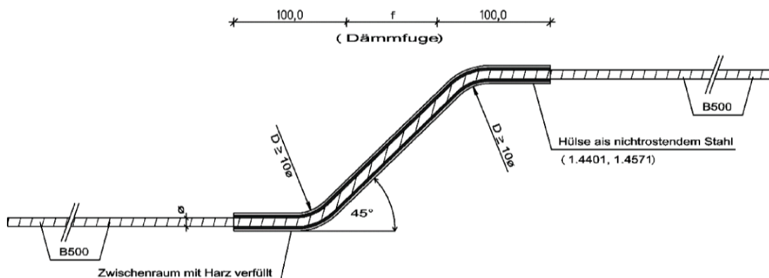
Abb. 17: Querkraftstabvariante 1
