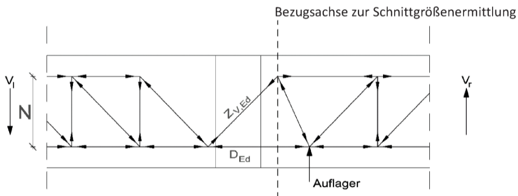
Abb. 39: Egobox Typ PV (statisches System)
