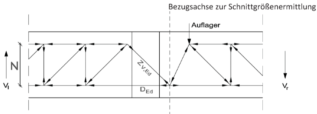
Abb. 41: Egcobox Typ PV± (statisches System)
