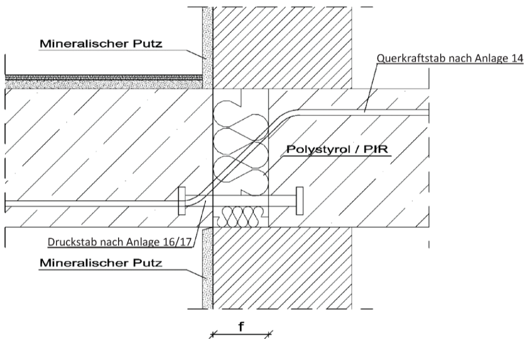
Abb. 35: Egibox Typ PV (Brandschutz)
