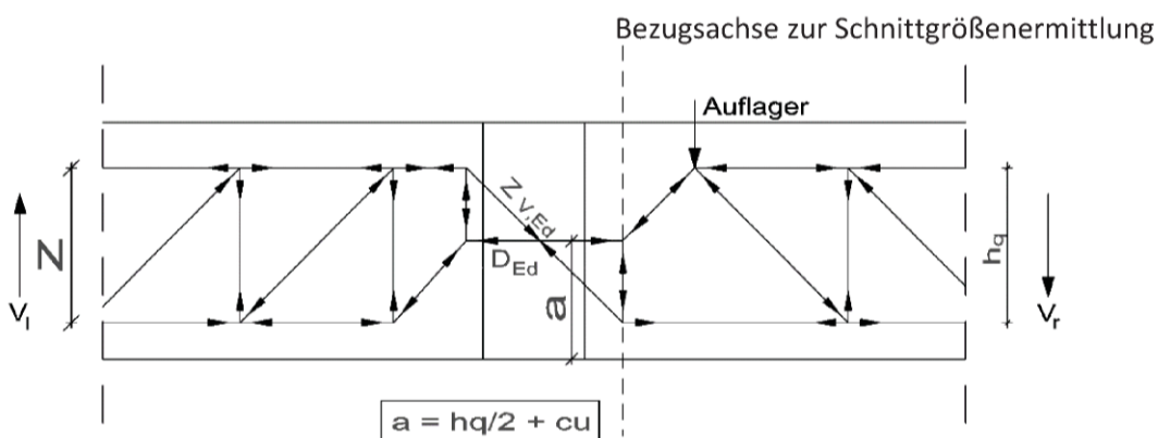
Abb. 42: Egcobox Typ PV± - mittiger Druckstab (statisches System)
