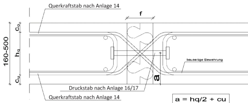
Abb. 7: Egcbbox Typ PV – mittiger Druckstab
