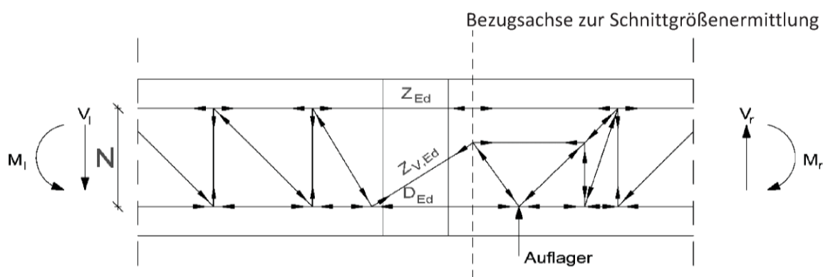
Abb. 37: Egcobox Typ P-F (statisches System)
