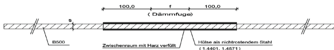
Abb. 20: Druckstabvariante 1
