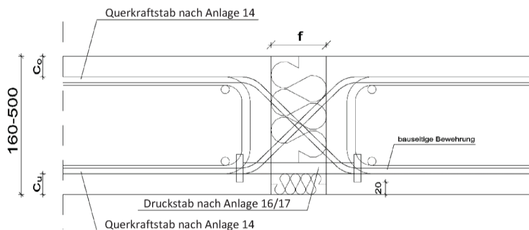
Abb. 6: Egcbbox Typ PV±
