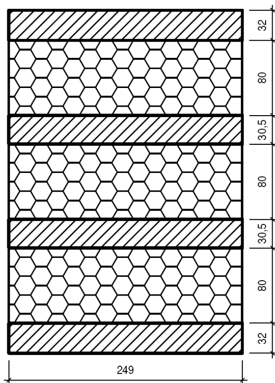
Schnitt B-B
