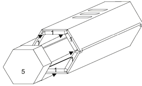
Rauchgasabdichtung aus 4 cm dicken „EasyFoam-Schaumstopfen“ oder „Sonifoam-Schaumstopfen“
