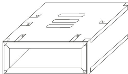
Montagelaschen
