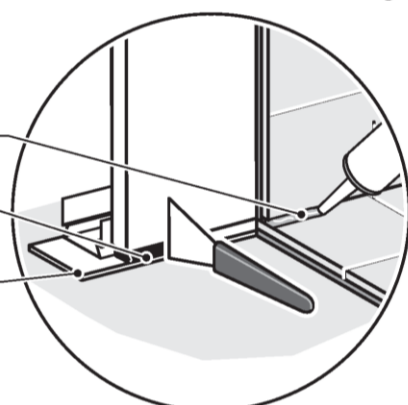
Anschluss Duofix Systemwand mit Fliesenbelag an Fußboden mit Fliesenbelag
