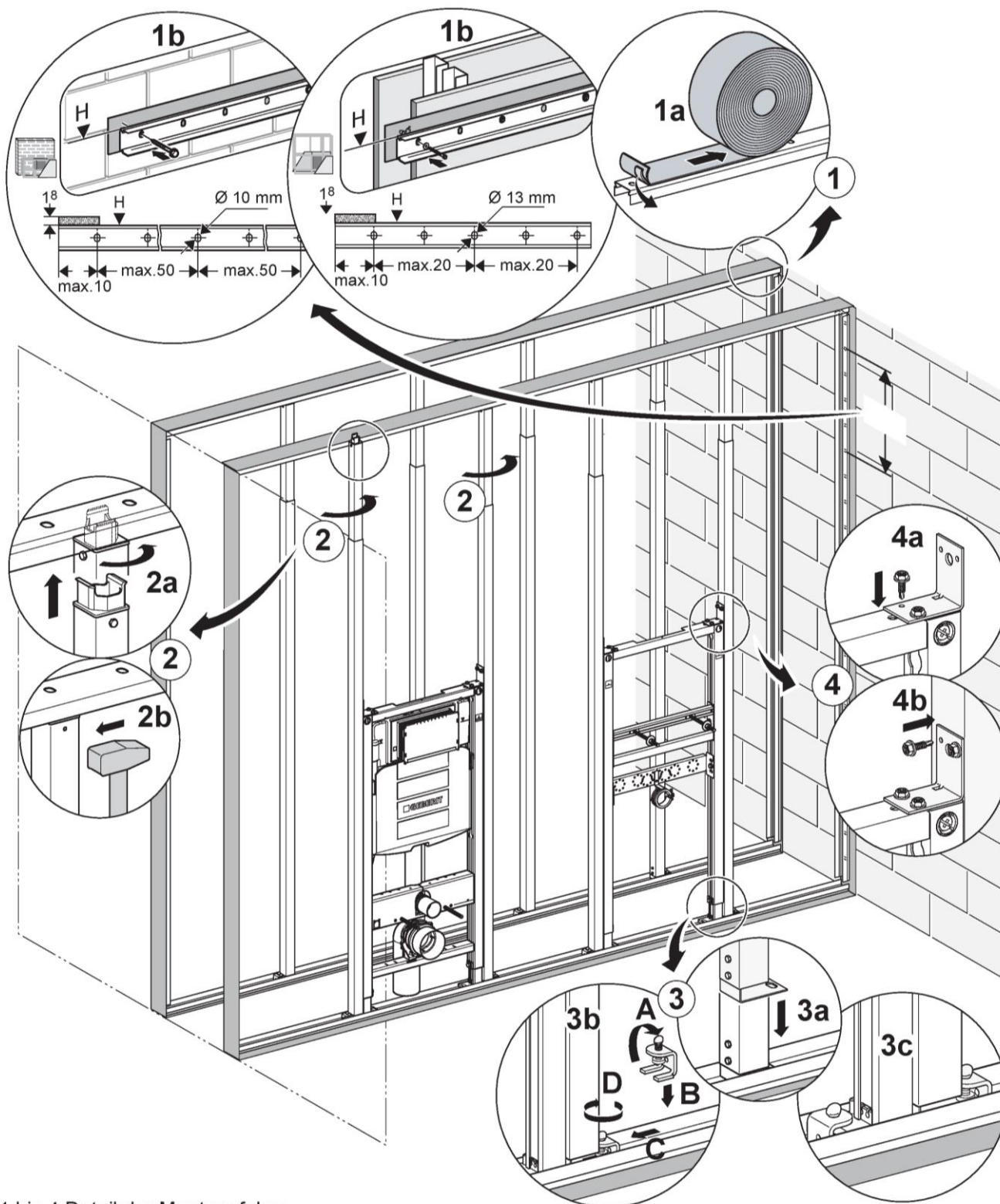
1 bis 4 Detail der Montagefolge
