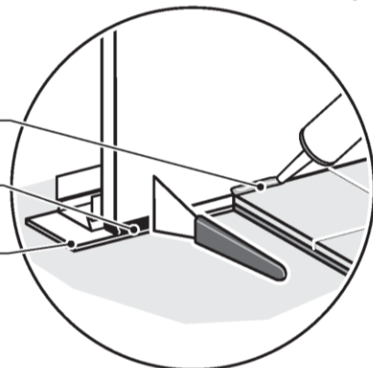
Anschluss Duofix Systemwand ohne Fliesenbelag an Fußboden mit Fliesenbelag
