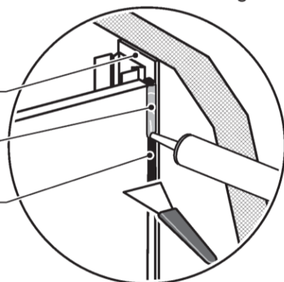
Anschluss Duofix Systemwand ohne Fliesen- belag an Massivwand ohne Fliesenbelag
