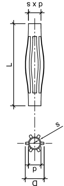
Federkorbbastabstandhalter
