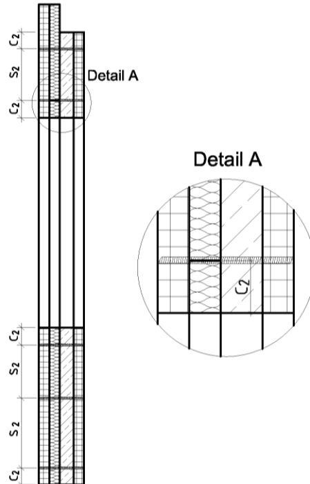
Schnitt B-B Elementwand:
