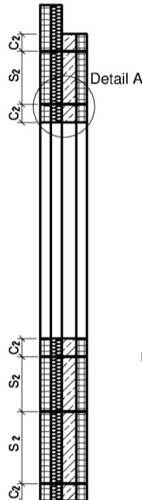
Schnitt B-B Elementwand:
