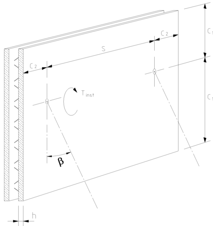
Bild 7: Mindestabstände, Neigungswinkel \beta der Stütze
