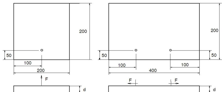
Bild 2: zentrischer Zug bzw. Querzug für einen Randabstand 50/100 mm
