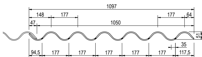
Bild 2: P6 mit 6 Wellen
