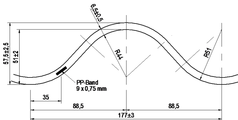
Bild 3: Maße und Lage des PP-Bandes
