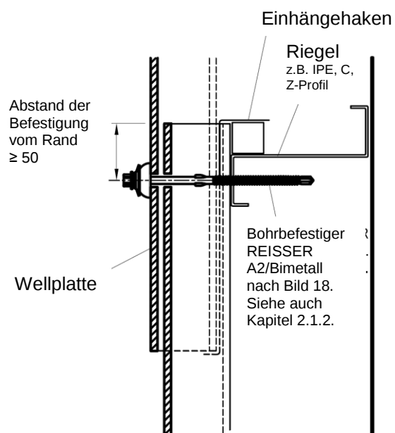
Bild 17b: Anordnung der Befestigungen auf dem Wellenberg bei Metall-UK
