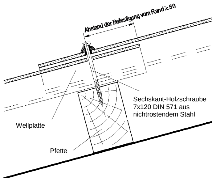
Bild 6: Anordnung der Befestigungen bei Holzpfetten
