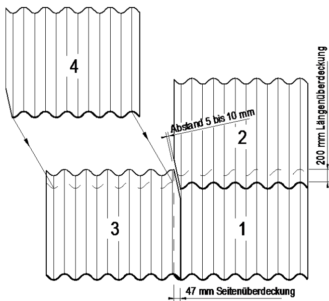
Bild 4: Überdeckungen und Eckenschnitte der Platte P5 und P6 Die Nummerierung der Wellplatten (1 bis 4) Kennzeichnet die Reihenfolge bei der Verlegung
