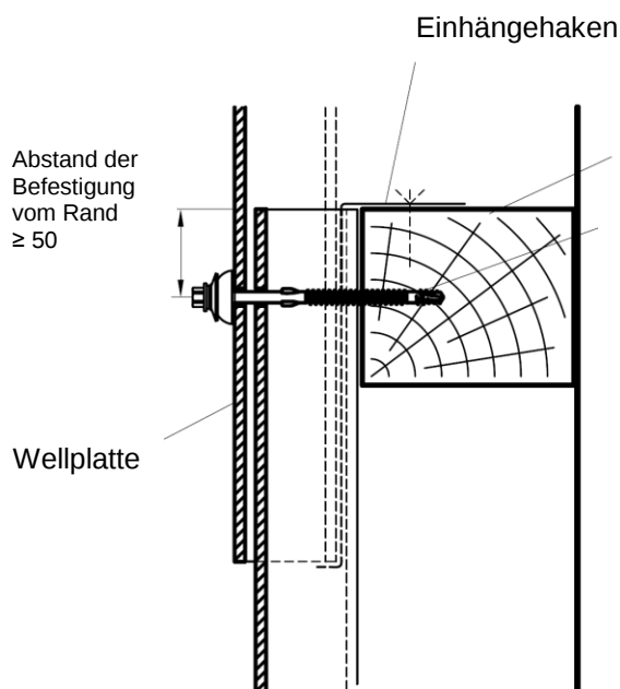
Bild 17a: Anordnung der Befestigungen auf dem Wellenberg bei Holz-UK
