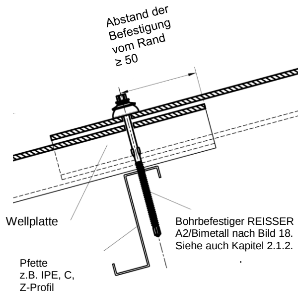
Bild 5b: Anordnung der Befestigungen bei Stahlpfetten mit Bohrbefestigung
