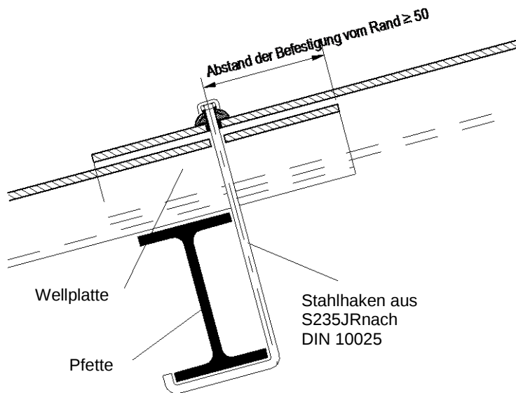
Bild 5a: Anordnung der Befestigungen bei Stahlpfetten
