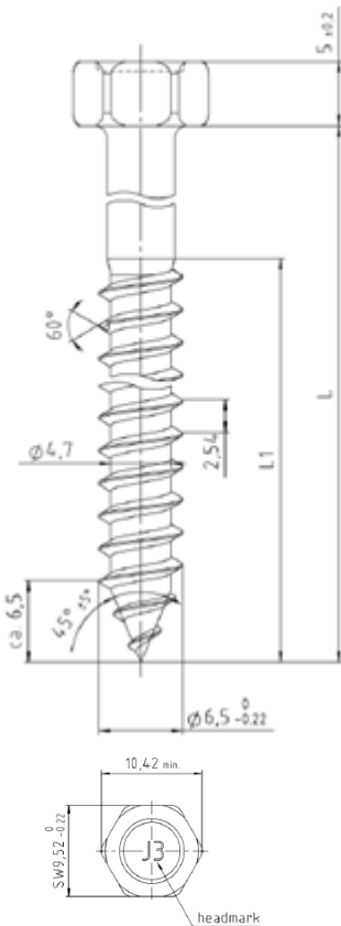
Bild 4b: Befestiger EJOT JA3-6,5 x L für Holzpfetten
