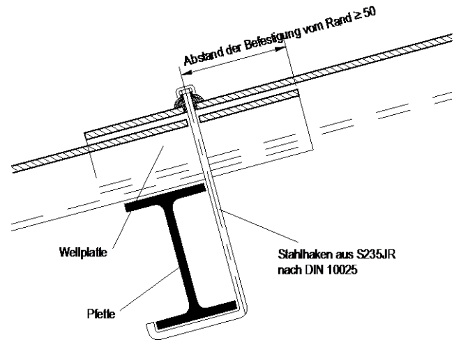
Bild 5: Anordnung der Befestigung auf Stahlpfetten
