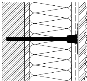
Dübelung gemäß Punkt 4.6.5
