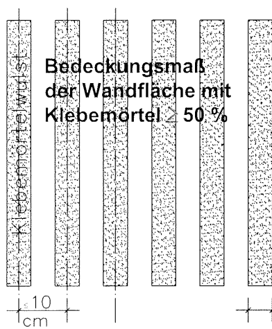
Teilflächenverklebung gemäß Punkt 4.6.4
