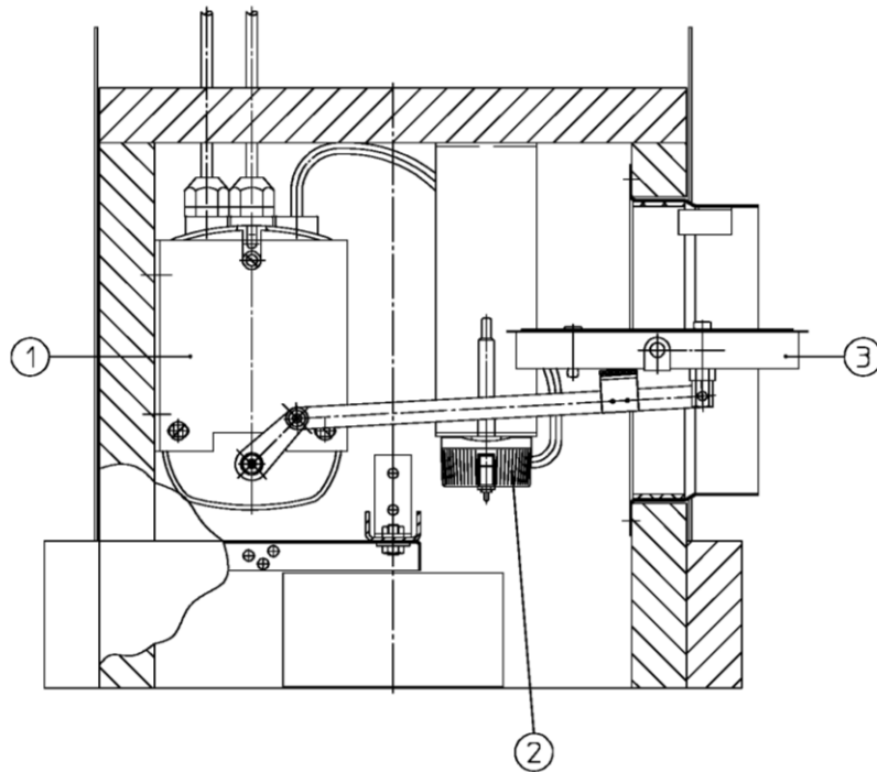
gez. Absperrklappe in AUF-Stellung
