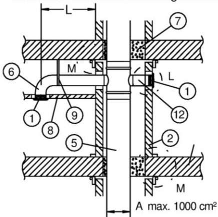
Einbau in feuerwiderstandsfähigen Schacht F30 - F90
