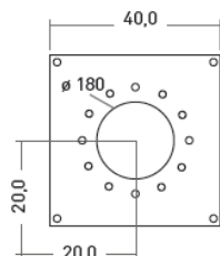
Frischluftzufuhr (unten)
