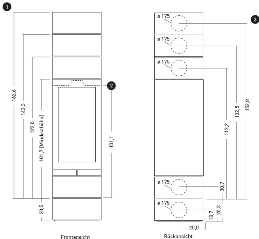
Rauchrohrabgang (oben)
