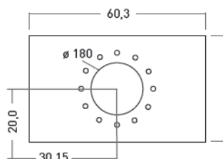
Frischluftzufuhr (unten)
