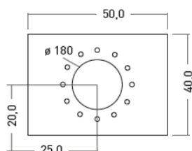
Frischluftzufuhr (unten)
