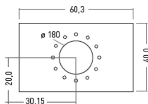
Frischluftzufuhr (unten)
