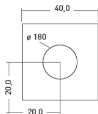
Rauchrohrabgang (oben)
