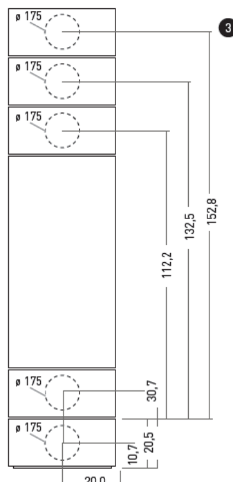
Seitenansicht
