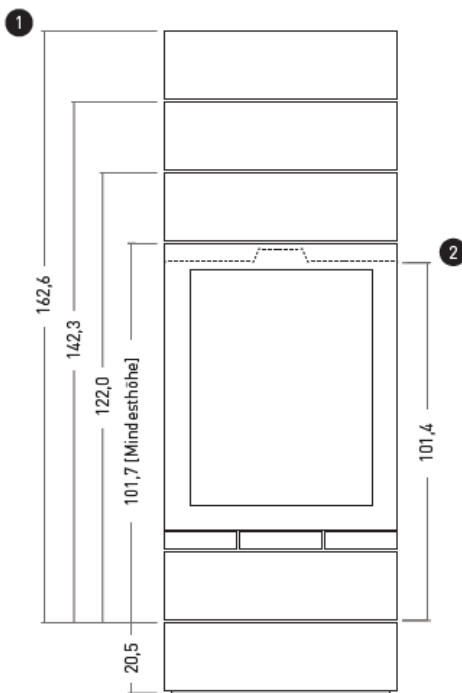
Frontansicht
