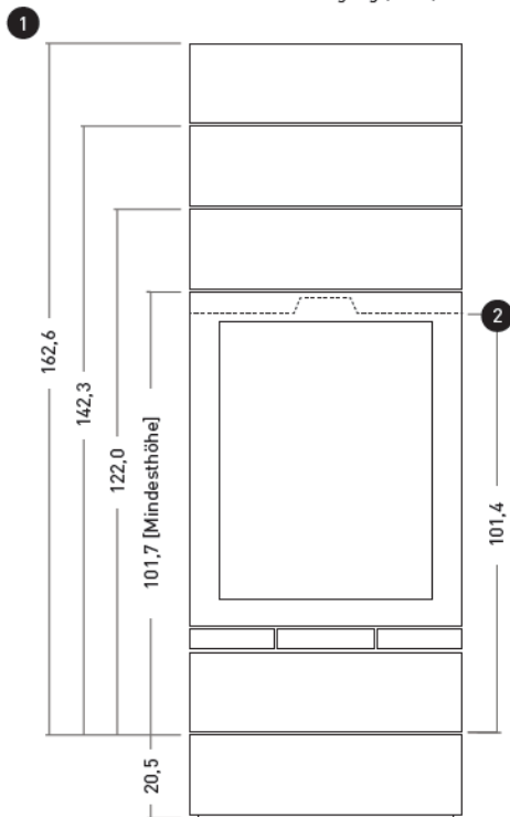
Rauchrohrabgang (oben)
