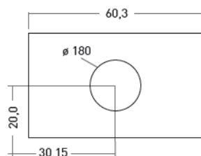
Rauchrohrabgang (oben)
