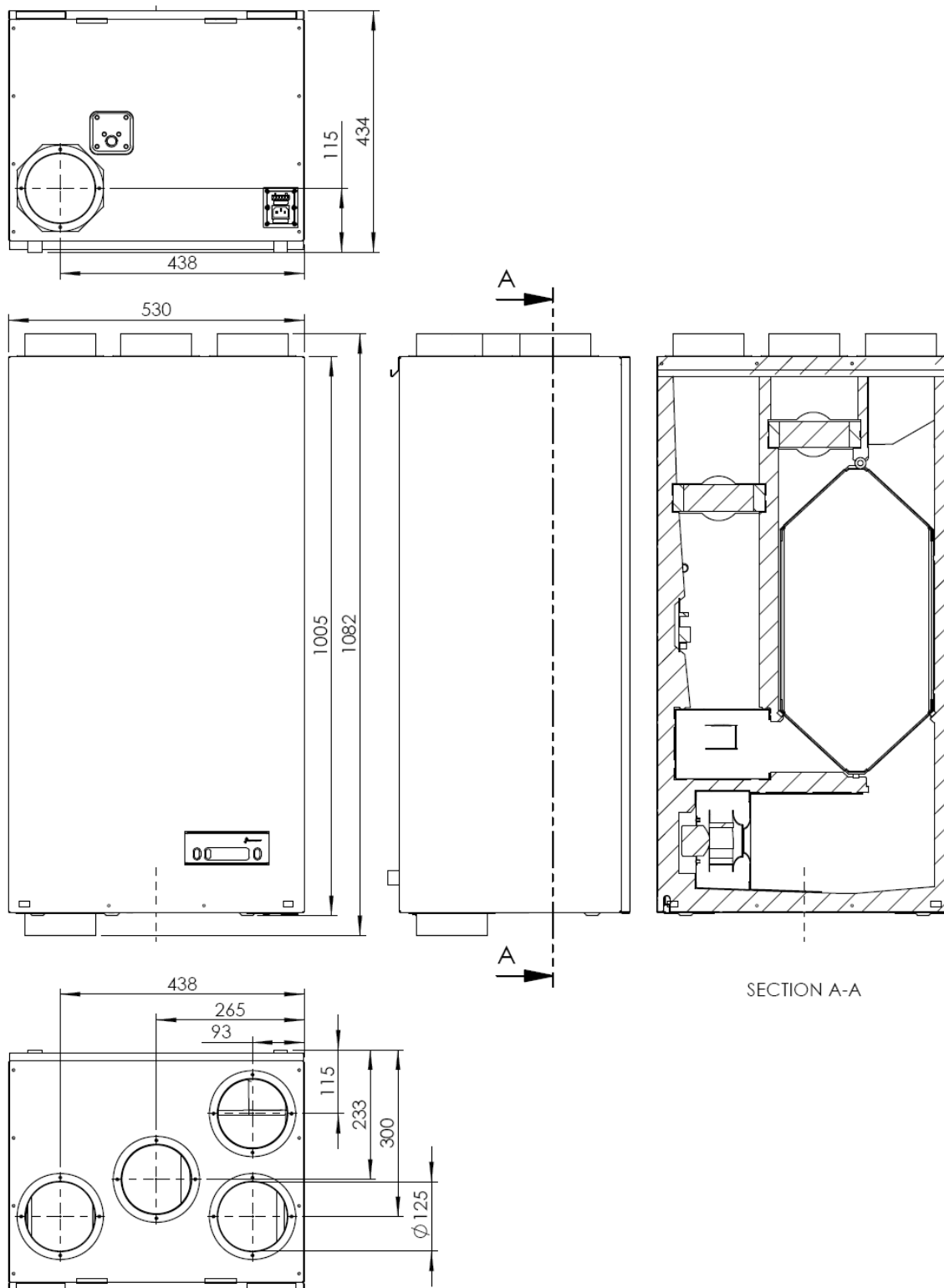
Maßangaben in mm
