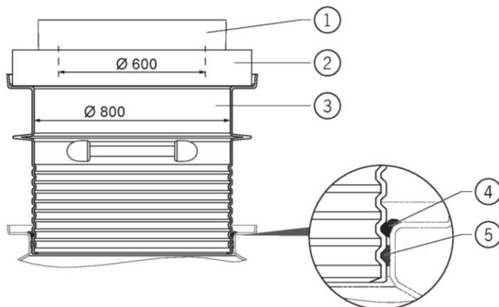
Abb.: Lastklasse E1 und E2 gemäß E DIN 19901
