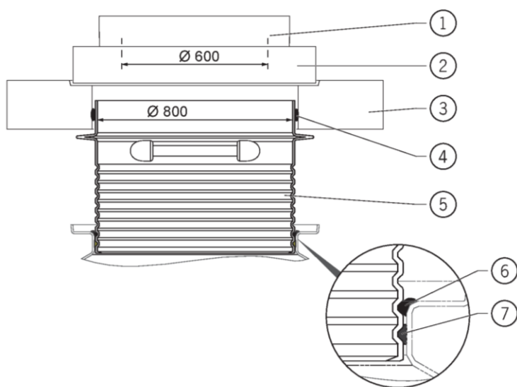
Abb.: Lastklasse E4 gemäß E DIN 19901
