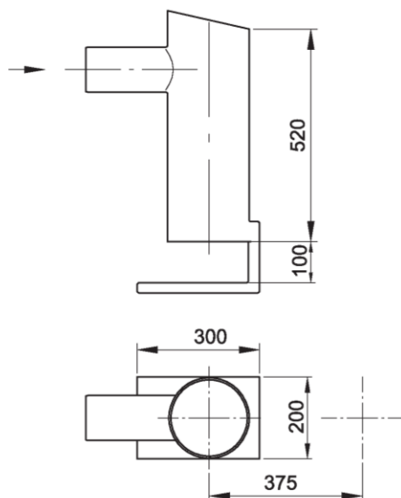
Abb.: NS 2 und 4
