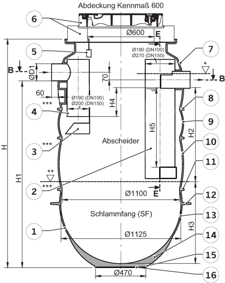
Abb.: Schnitt A-A
