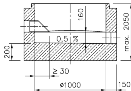
Probenahmeschacht
