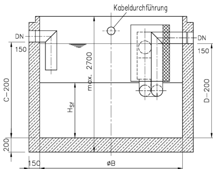
Abscheider Kl. II u. I mit integriertem Schlammfang
