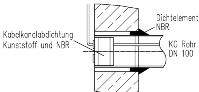
Kabeldurchführung für Warnanlage
