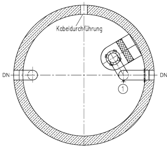
Kabeldurchführung für Warnanlage
