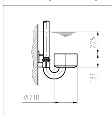
Ölabsaugevorrichtung
