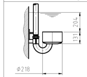
Ölabsaugevorrichtung
