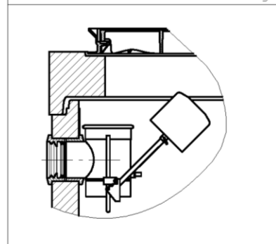
Zulaufausführung für Option Zulaufsperrung (Zusatzverschlußeinrichtung)
