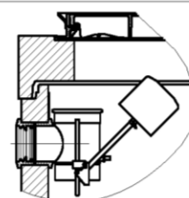
Zulaufausführung für Option Zulaufsperrung (Zusatzverschlußeinrichtung)
