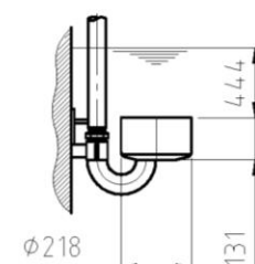
Ölabsaugevorrichtung
