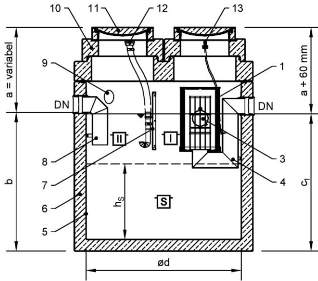
Ausführung mit Probenahmereinrichtung [S II I P]
