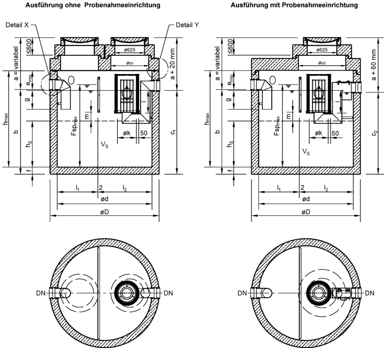
Schachtaufbau: DIN EN 1917 in Verbindung mit DIN V 4034-1 Typ 2, Zugänglichkeit nach DIN EN 476
