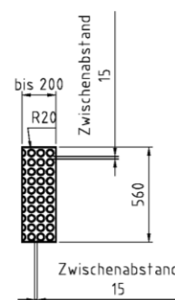
Detail Koaleszenzgitter
