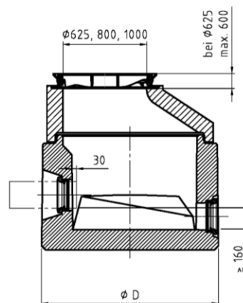
Probenahmeschacht als Probenahmeverrichtung gemäß DIN 1999-100
