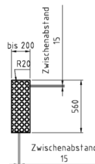
Detail Koaleszenzgitter
