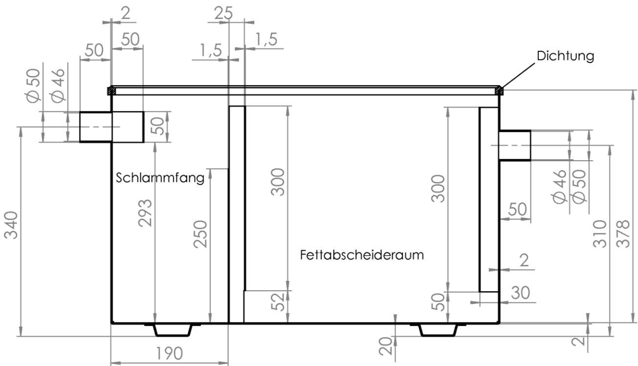
Schnitt B-B M1 : 6
