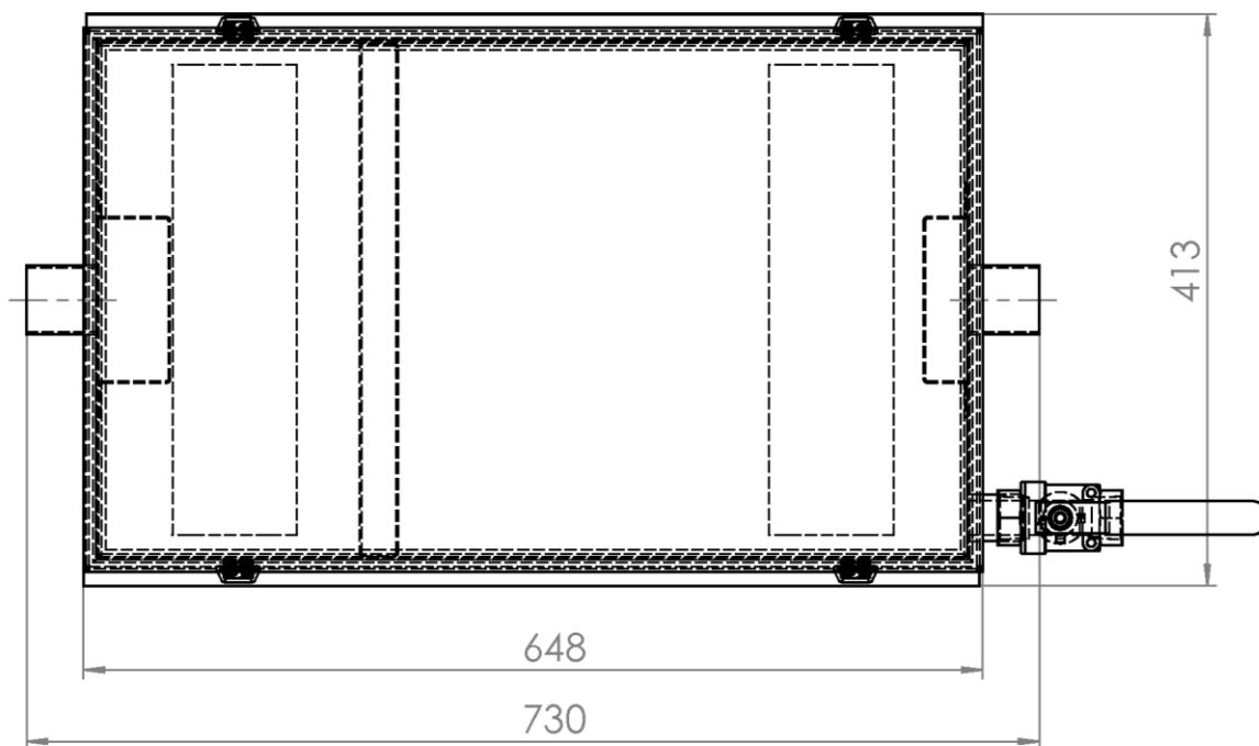
Draufsicht M 1:6
