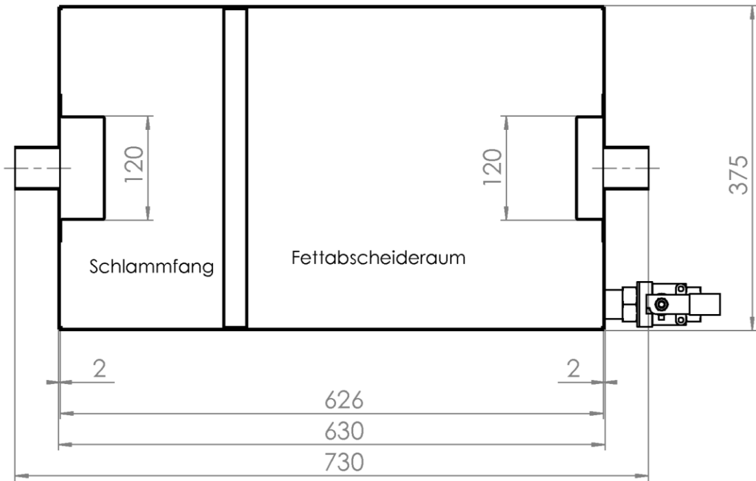
Schnitt A-A M1 : 6
