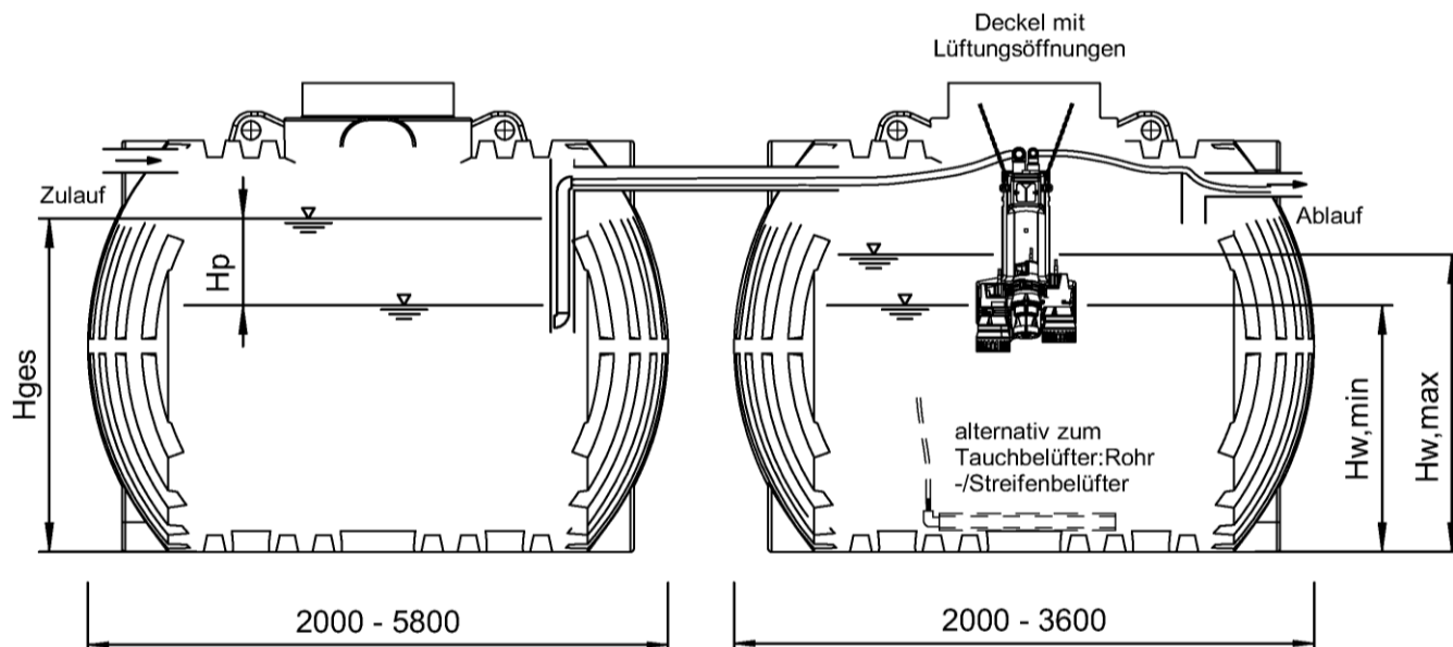
Grobfang / Schlammsp.
