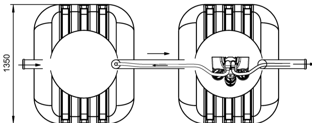
Grobfang/ Schlammsp.
