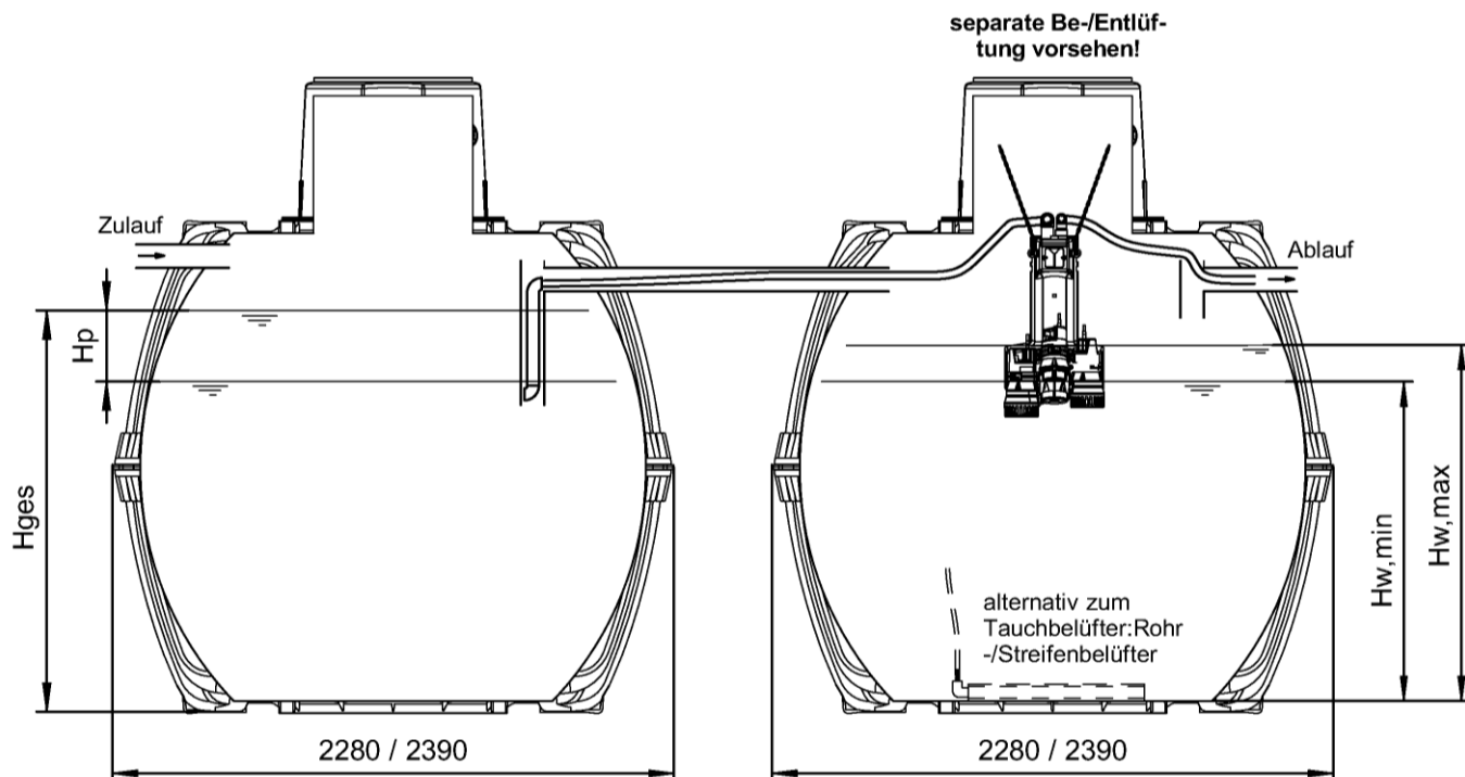
Grobfang / Schlammsp.
