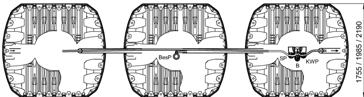
Belebungs / SBR
