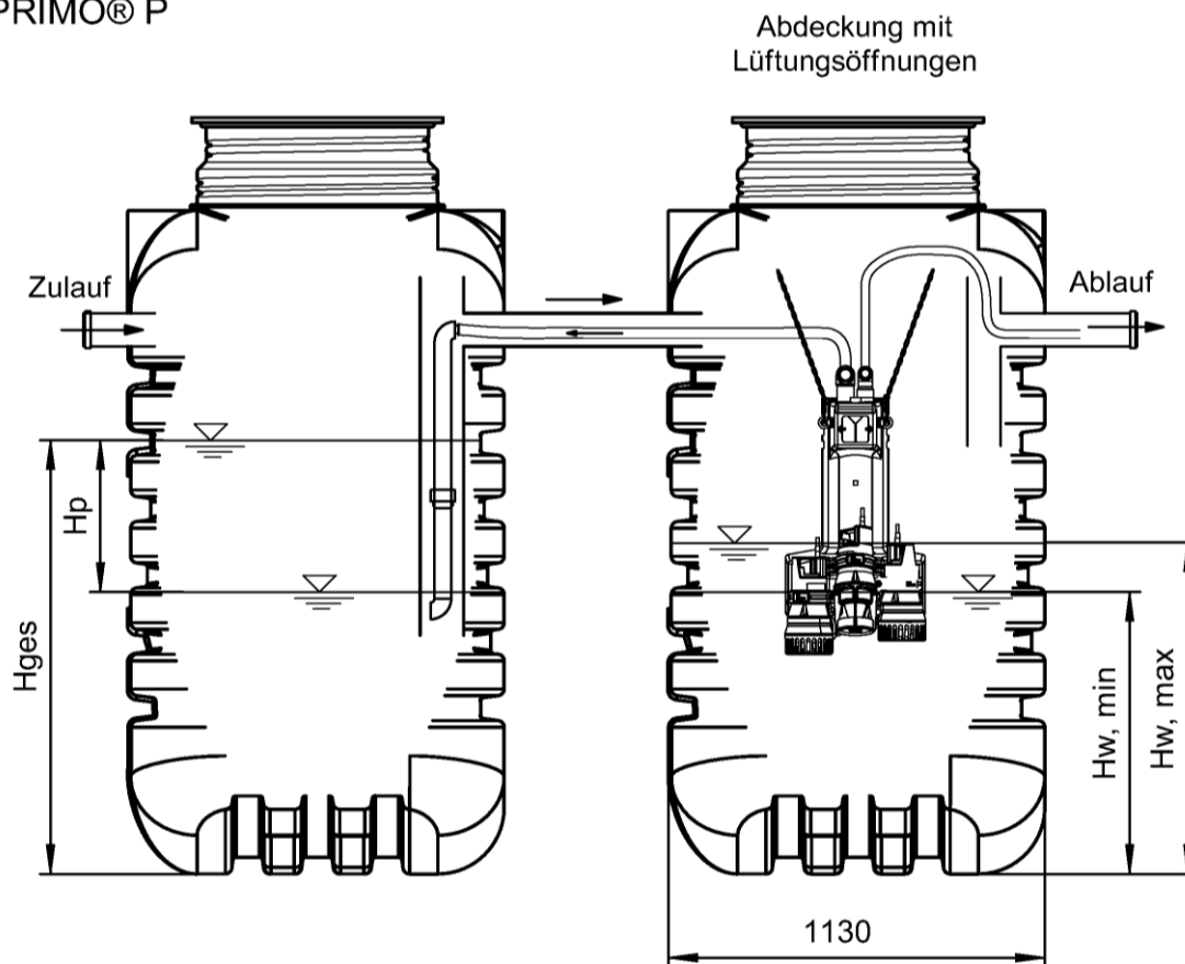
Grobfang/ Schlammsp.
