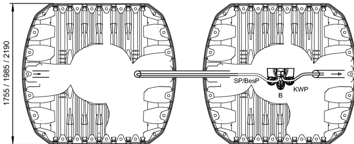
Belebungs SBR
