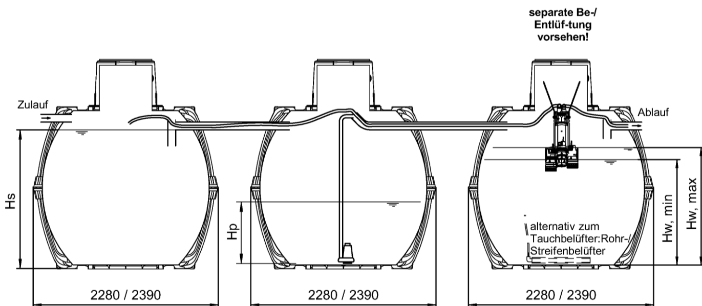
Grobfang / Schlammsp.
