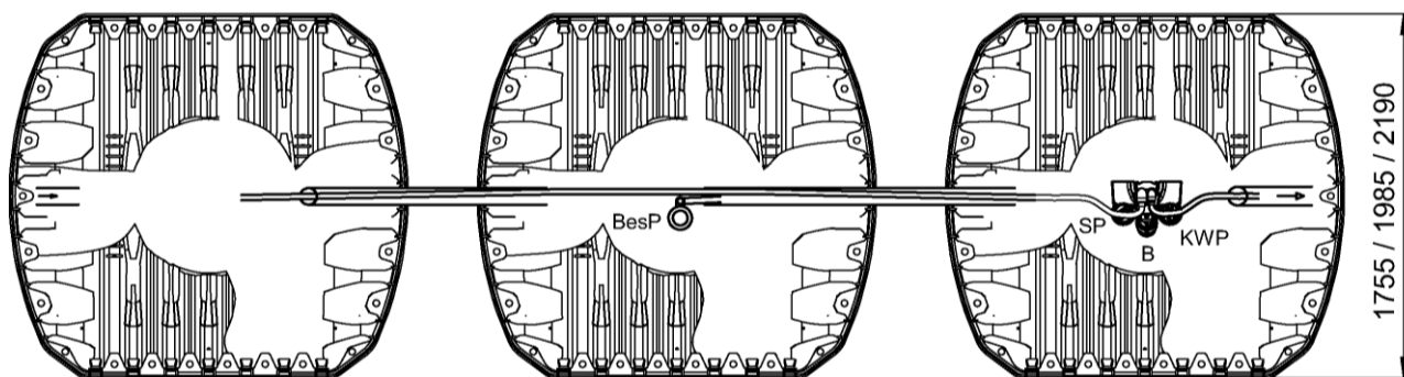
Belebung / SBR
