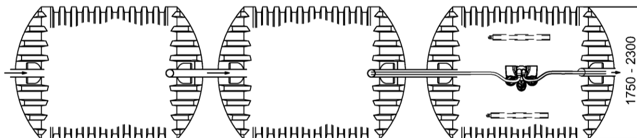
Grobfang / Schlammspeicher
