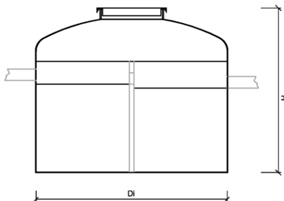
Konusabdeckung
