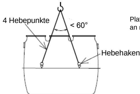
Position der Hebegurte
