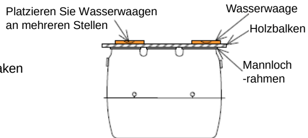
Ausrichten der Anlage
