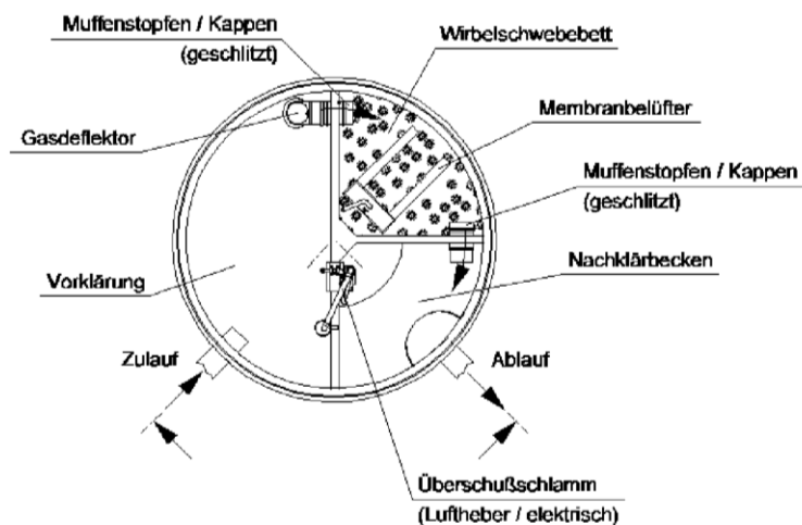
Draufsicht ohne Abdeckung
