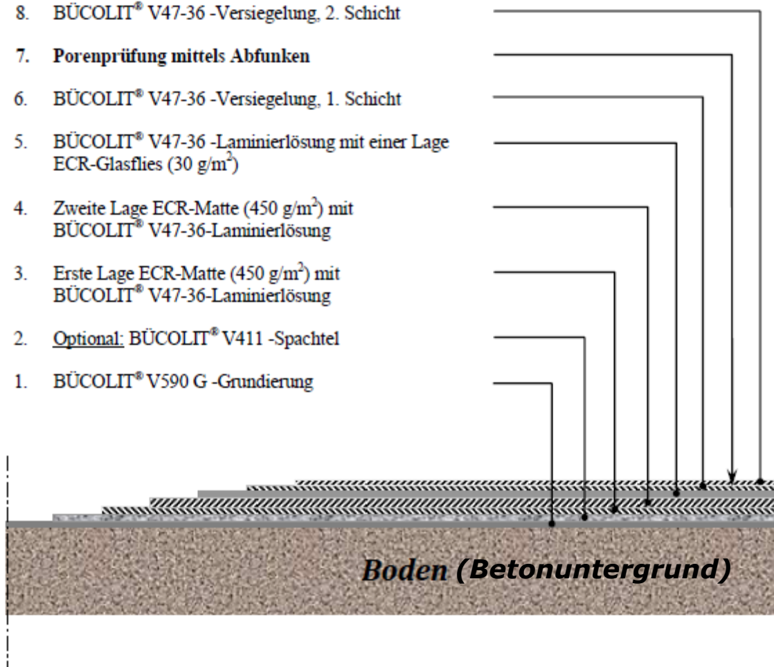
Beschichtungsaufbau auf dem Betonuntergrund (Boden) gemäß Abschnitt 3 der Zulassung
