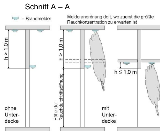
Bild 1: Maßgebende Höhe der Deckenunterfläche
