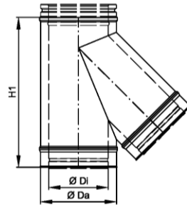
Rauchrohranschluss 45°
