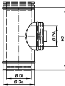
Putztüranschluss (Überdruck)
