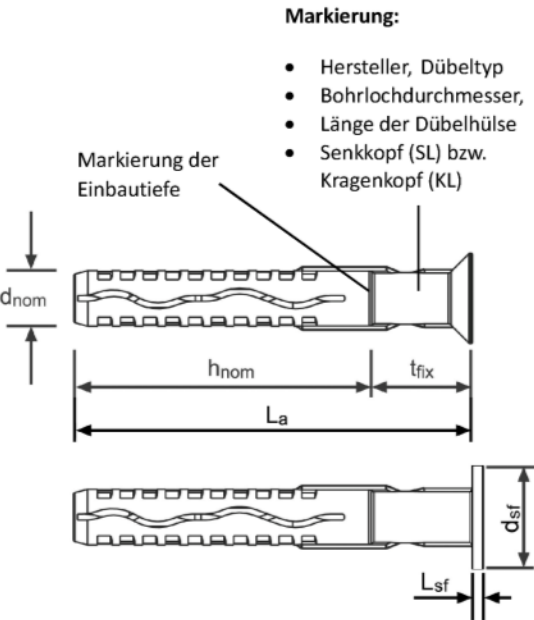
Dübelhülse KT 14
