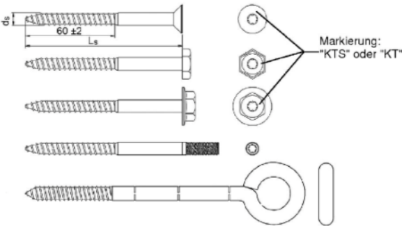
Spezialschraube KT 14
