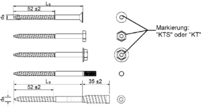
Spezialschraube KT 14
