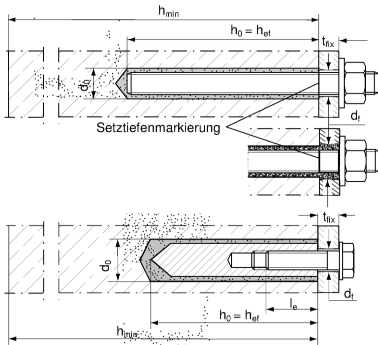
Ankerstange Vorsteckmontage
