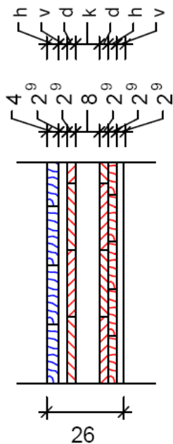
Wandtyp 26 horizontal
