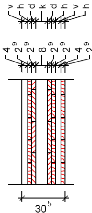
Wandtyp 30,5 vertikal
