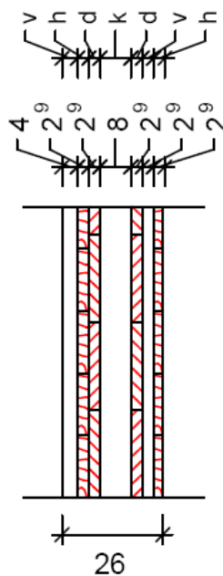
Wandtyp 26 vertikal
