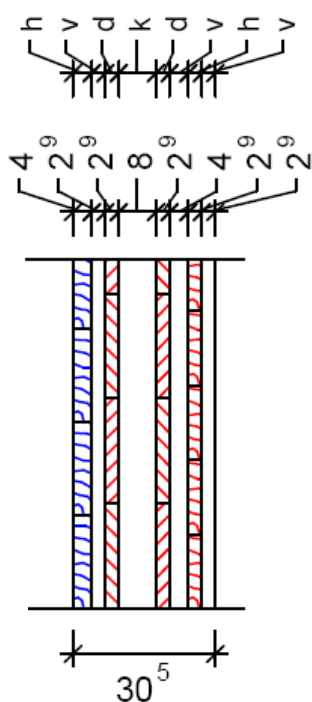
Wandtyp 30,5 horizontal
