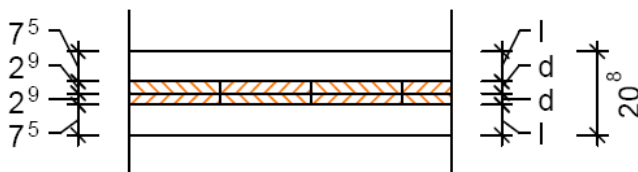
Längsschnitt 2
