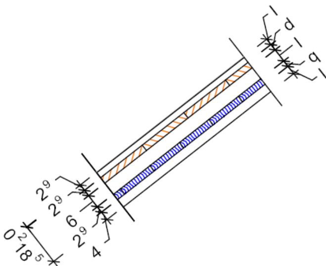
Dachtyp 18,5
