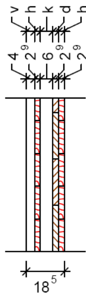
Wandtyp 18,5 vertikal
