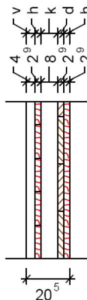
Wandtyp 20,5 vertikal
