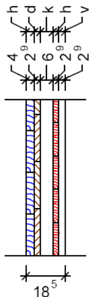
Wandtyp 18,5 horizontal
