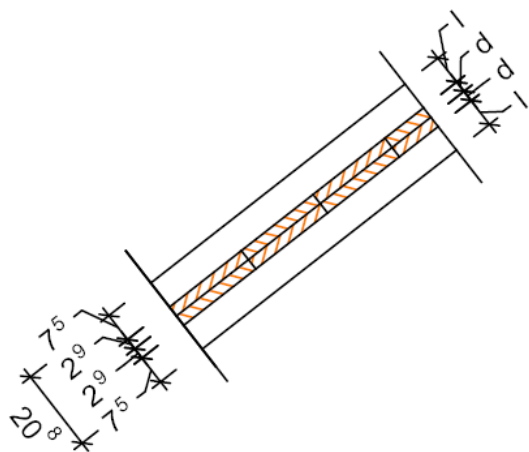
Längsschnitt 1
