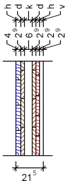
Wandtyp 21,5 horizontal
