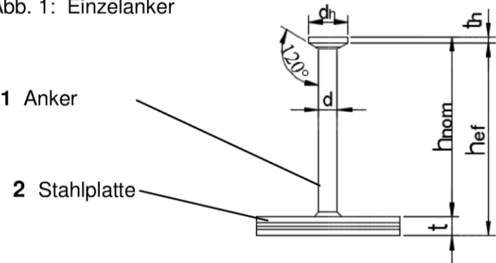
Abb. 1: Einzelanker
